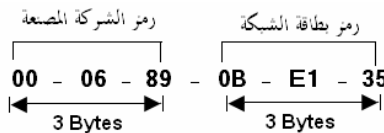
شكل ٢-٥ تنسيق العنوان المادي
