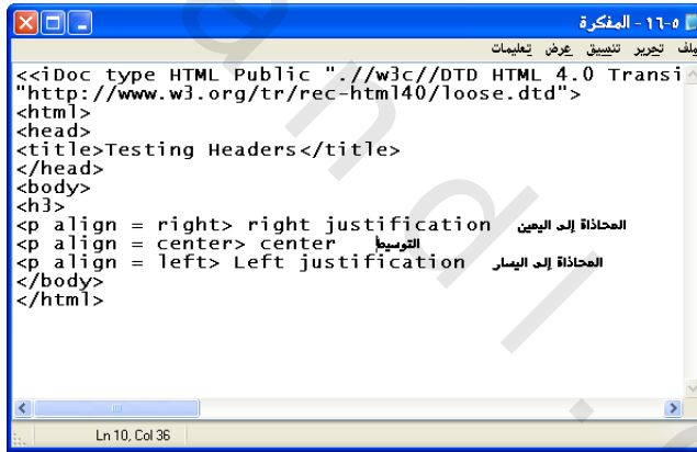
شكل ١٦-٩ برنامج بسيط لعرض عناصر محاذاة الفقرات
