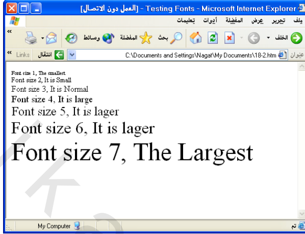
شكل ١٨-٢ استخدمنا الأحجام المتاحة في العنصر Size
