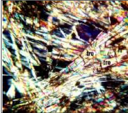
شكل (٧٧) عينة من حجر السربنتنايت تحت الميكروسكوب توضح النسيج المميز له والمكونات
