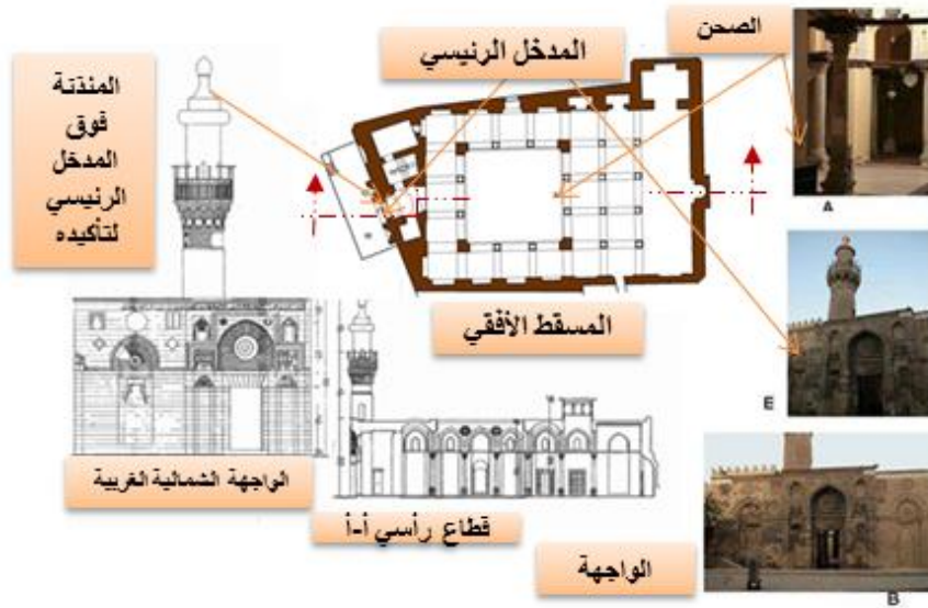
شكل (١٢/٢/١): مسجد الأقمر ٥١٩ هـ : مسقط أفقي - قطاع رأسي أ-أ - واجهة شمالية غربية.
