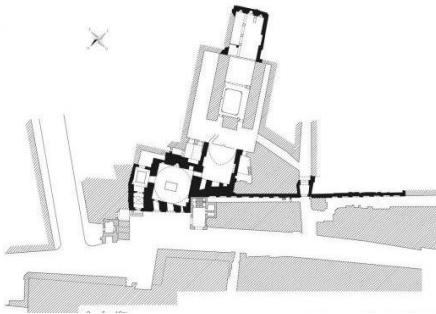
شكل (١٦/٢/١): المدرسة الصالحية - المسقط الأفقي.
