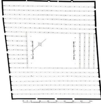
شكل (١/٢/١): مسجد عمرو بن العاص - المسقط الأفقي للجامع حالياً.
