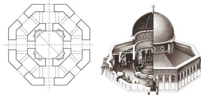
شكل (٣٥/٢/١): مقطع منظوري في قبة الصخرة / مسقط أفقي لضريح الصليبية .
