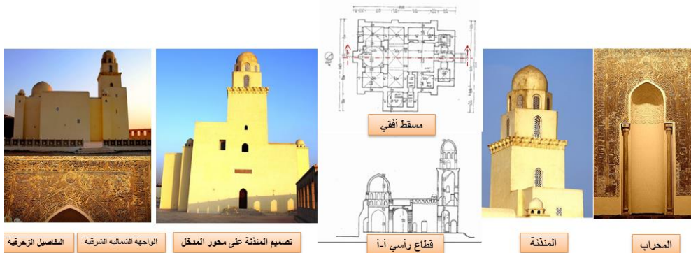
شكل (١٤/٢/١) : مسجد الجيوشي - المسقط الأفقي - الواجهة الشمالية الشرقية - التفاصيل المعمارية.
