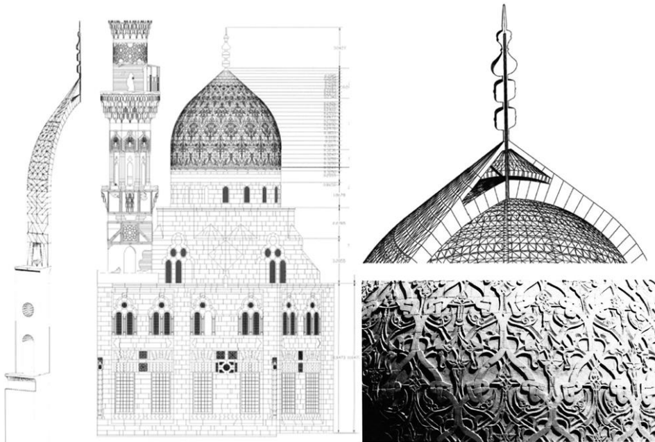
شكل (٢٣/١/٢): قبة مدرسة الأمير خاير بك ١٥٠٢م: قطاع رأسي يوضح الهيكل البنائي للقبة – تفاصيل القبة الزخرفية- الواجهة وشكل القبة من الخارج – وحدة من ٢٠ وحدة متكررة تتكون منها هيكل القبة .
