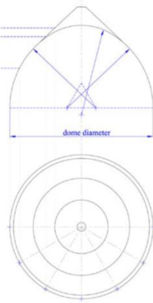
شكل (١٦/١/٢) : قطاع القبة البيضاوي الشكل لأحد القباب المملوكية .
