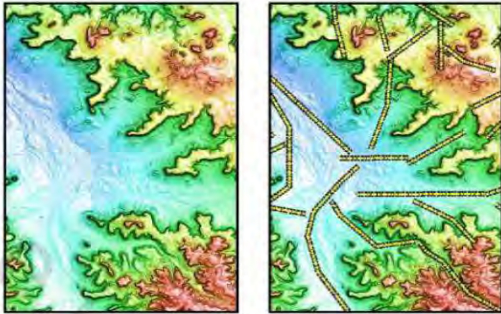
Figure 3.11. Stereo satellite elevation image. (Sandra et al, 2011)
