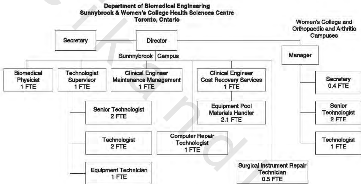
الشكل رقم (١٧,١). قسم الهندسة الإكلينيكية في مركز SWCHSC.
