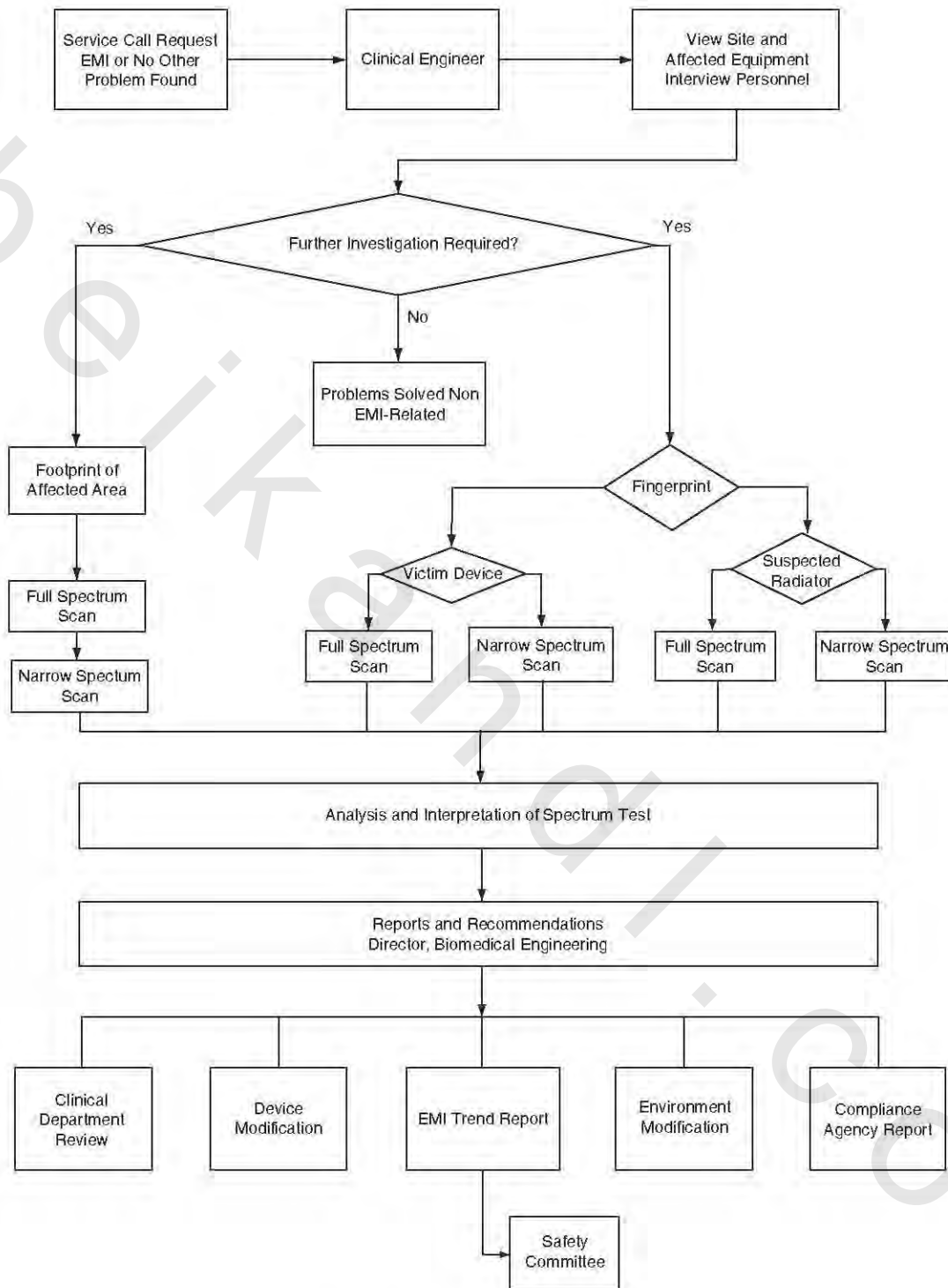
الشكل رقم (٢، ٦٣). مخطط جريان لحل مشكلة تداخل كهرومغناطيسي.
