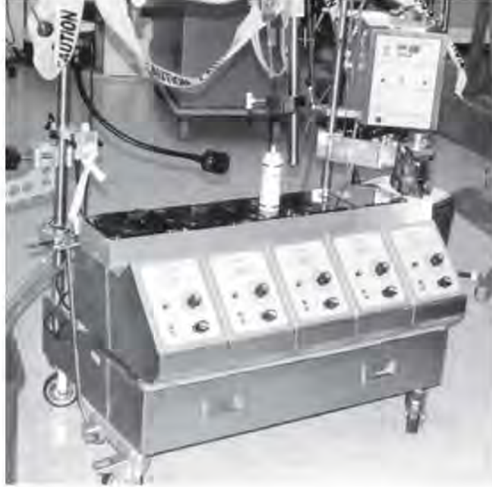
الشكل رقم (٨٩، ١٠). جهاز القلب-الرئة نوع Stockert-Shiley تحت التجريب في المختبر.
