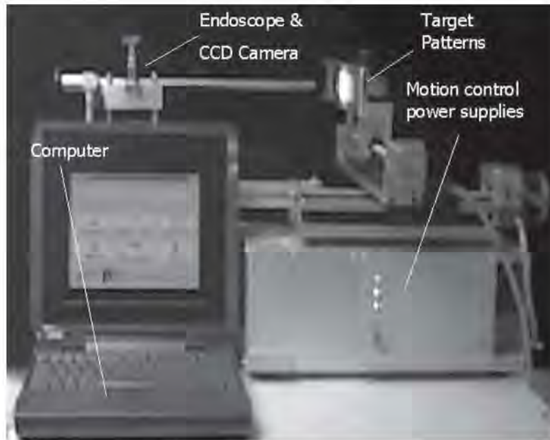
الشكل رقم (٩٢،٦). مُنْبَت الاختبار الأساسي للـ EndoTester TM .
