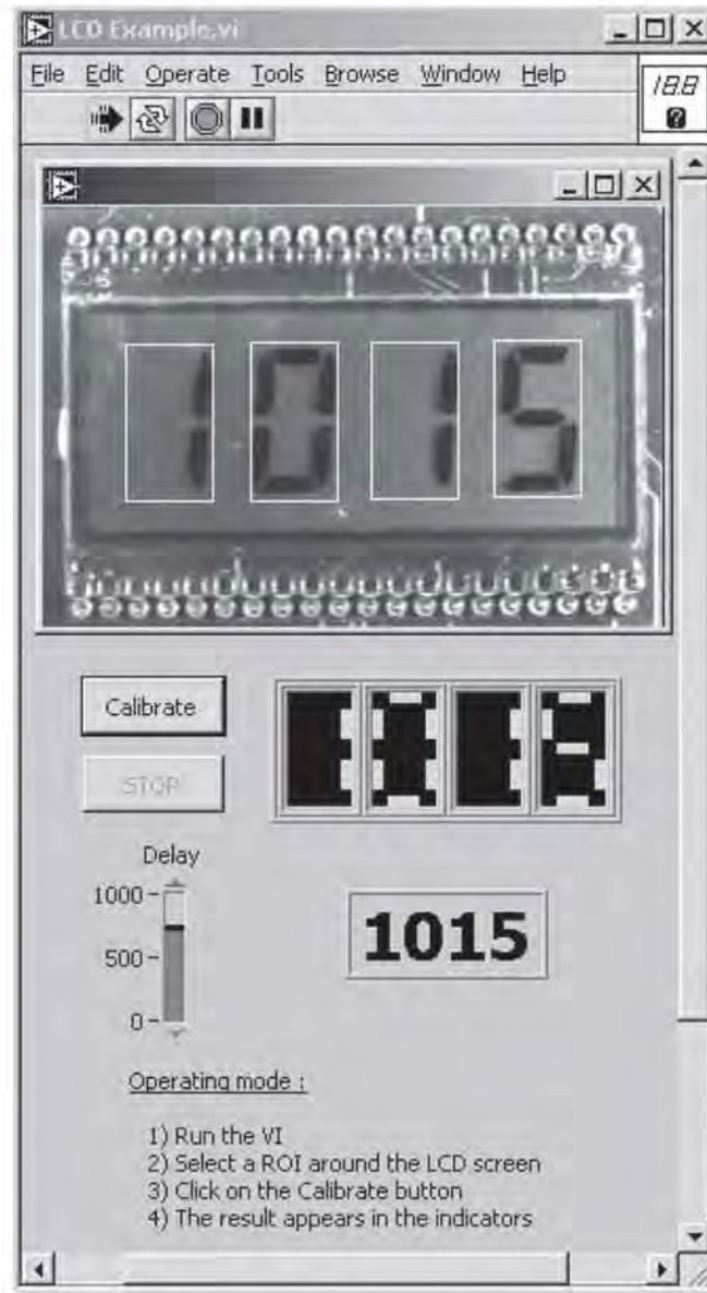
الشكل رقم (٢، ٩٢). مثال عن الإظهار بالكريستال المسائل (LCD) ذي القطع المسبعة.
