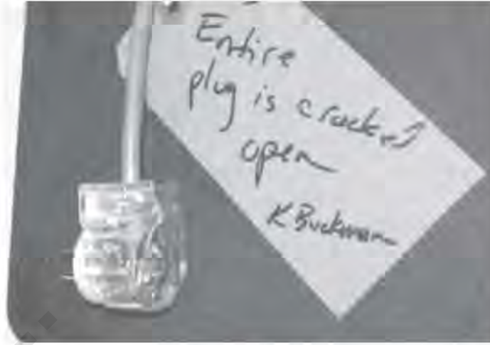
الشكل رقم (٧٦,٥). شقوق متعددة لوحظت في قابس سلك التغذية بالطاقة لمبخرة.
