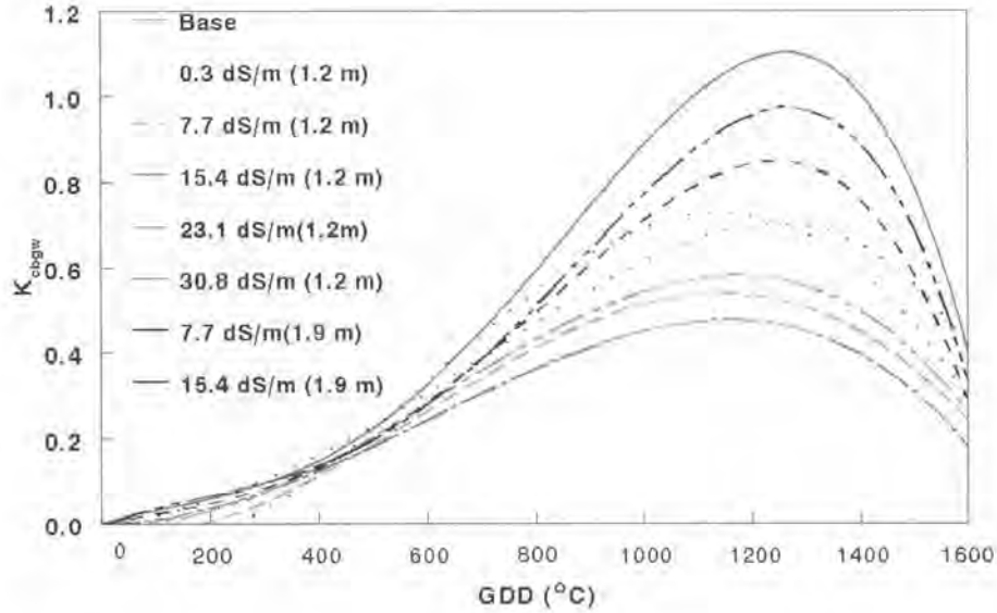
الشكل رقم (١٨،٧). معامل باسال لخصول القطن والمحسارات معاملات محصول المعدلة المشتقة من بيانات الليسوميترات لخمس كميات من المياه الجوفية عند أعماق مختلفة.
