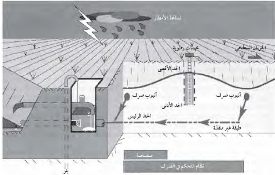
الشكل رقم (١٨، ١). نموذج للتحكم في الصرف والري التحقي عند تشغيل إدارة منسوب الماء الأرضي، التحكم في مستوى مصب المياه (غرفة التفريش) يعتمد على التغذية الراجعة لعمق منسوب الماء الأرضي في الحقل.
