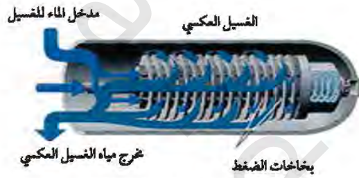
الشكل رقم (٢٥، ١٠). المرشح القرصي.
