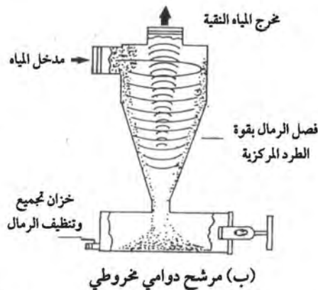
الشكل رقم (٢٤, ١٠). المرشح الدوامي (الطارد المركزي).
