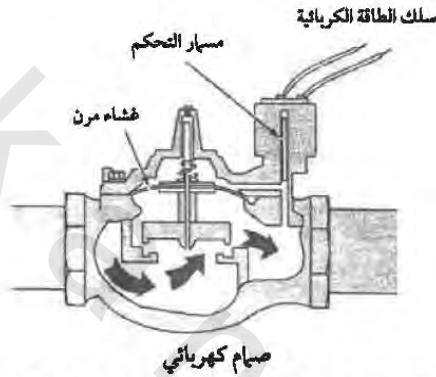
الشكل رقم (١٧، ١٠). الصمام الرئيس في مركز التحكم لنظام الري بالتنقيط.
