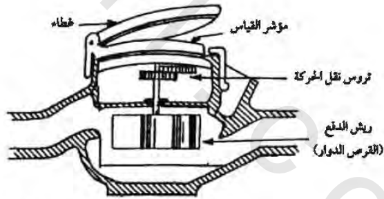
الشكل رقم (١٩ ، ١٠). العداد المروحي لقياس كمية المياه.
