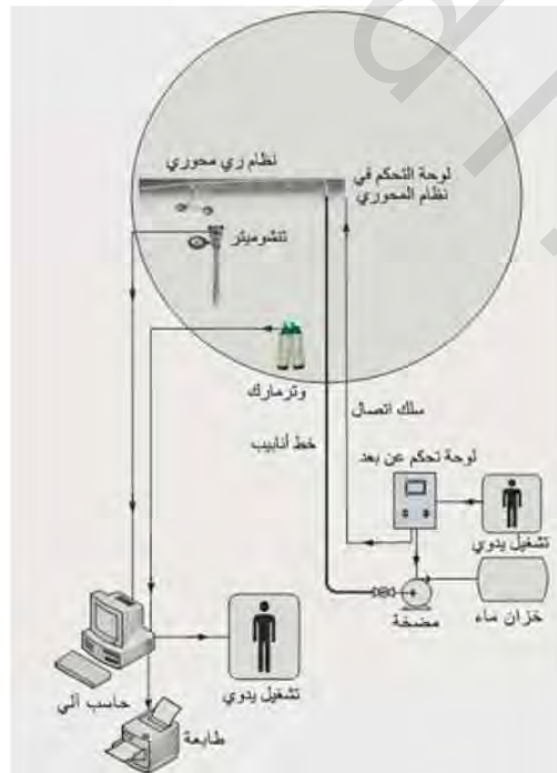
الشكل رقم (١٣، ١١). مخطط لمكونات الري الذكي الآلي ذو الدائرة المفتوحة باستخدام مجسات الشد الرطوبي.
