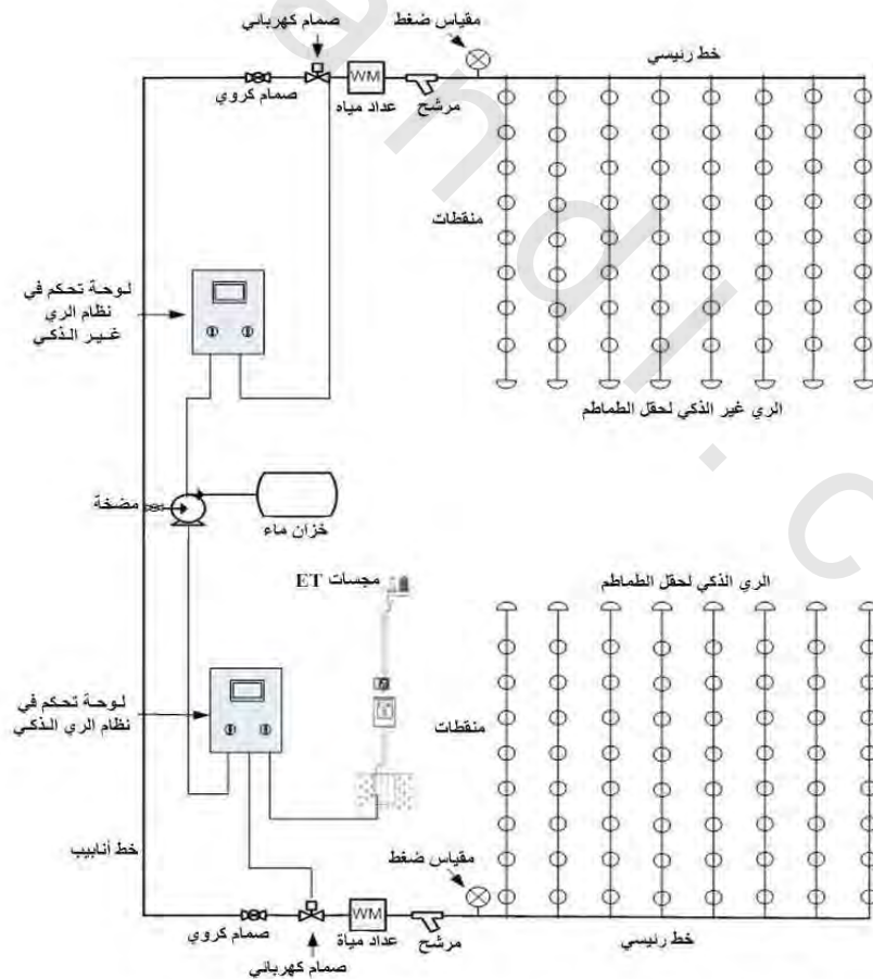
الشكل رقم (٨، ١١). وحدة التحكم الذكية مع نظام المري بالتنقيط.
