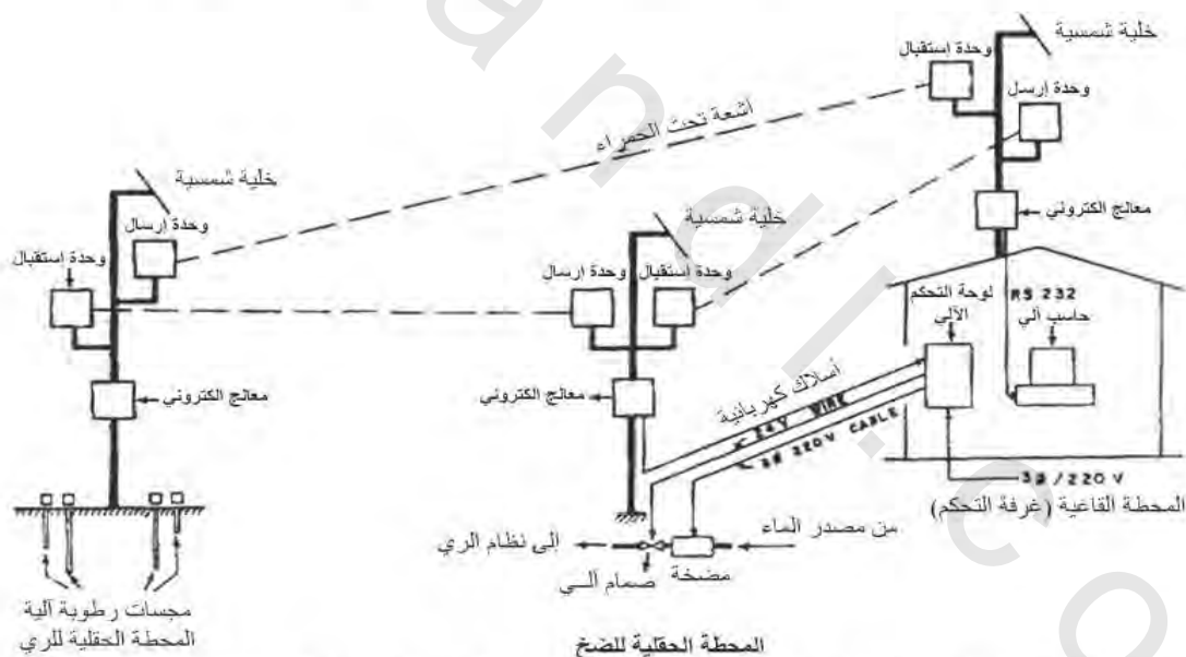
الشكل رقم (١١، ٣٦). استقبال وإرسال المعلومات من محطة التحكم إلى المحطة الحقلية بواسطة الأشعة تحت الحمراء.
