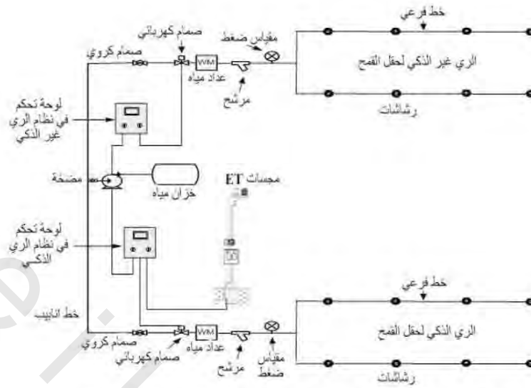
الشكل رقم (٧، ١١). وحدة التحكم الذكية مع نظام المري بالرش.
