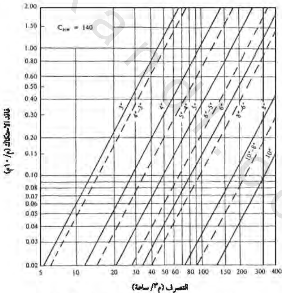
الشكل رقم (١٢، ٤). لفائد الاحتكاك عند تصريفات مختلفة وأقطار مختلفة.
