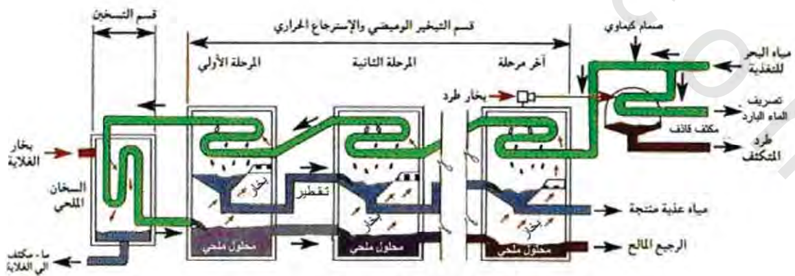
الشكل رقم (١٠، ١). تحلية مياه البحر بطريقة التبخير الوميضي.
