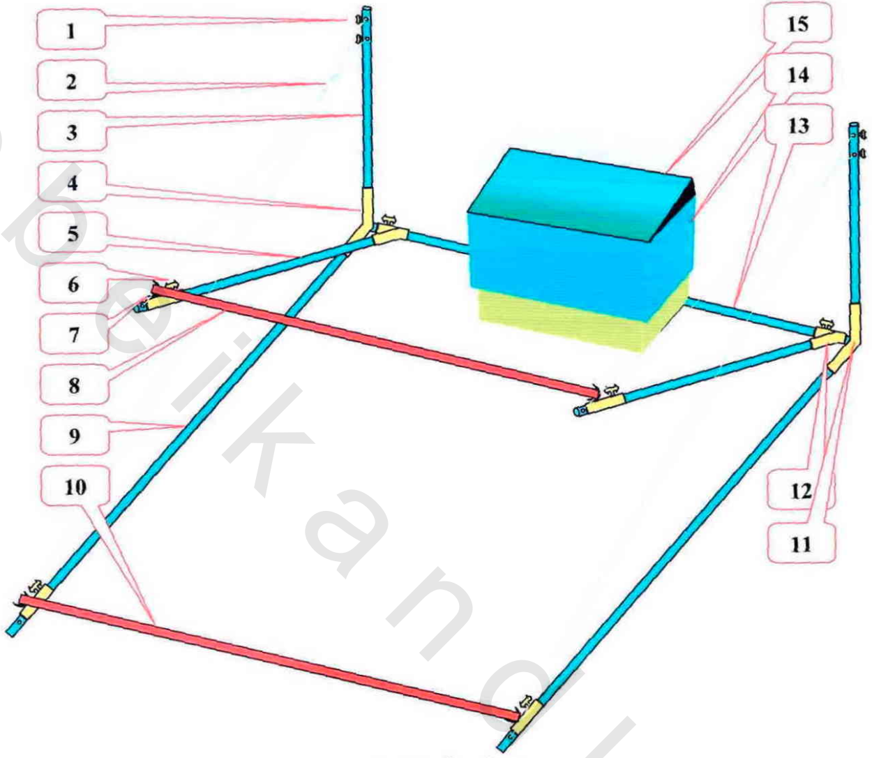
شكل رقم ( 22 ) الشكل النهائي لجهاز قوة الدفع الإضافي المطور
