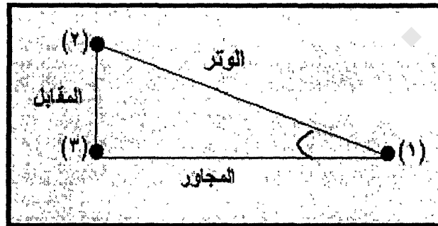
شكل رقم ( 23 ) مكونات المثلث قائم الزاوية
