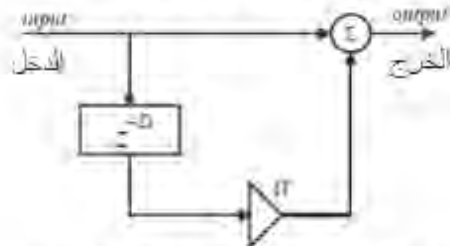
الشكل رقم (١٠.٩) - مرشح الصدى الأحادي
