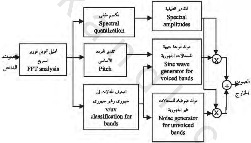
الشكل رقم (٢، ١٠). استخدام المكونات الطيفية لإشارة الصوت في تشفيره.
