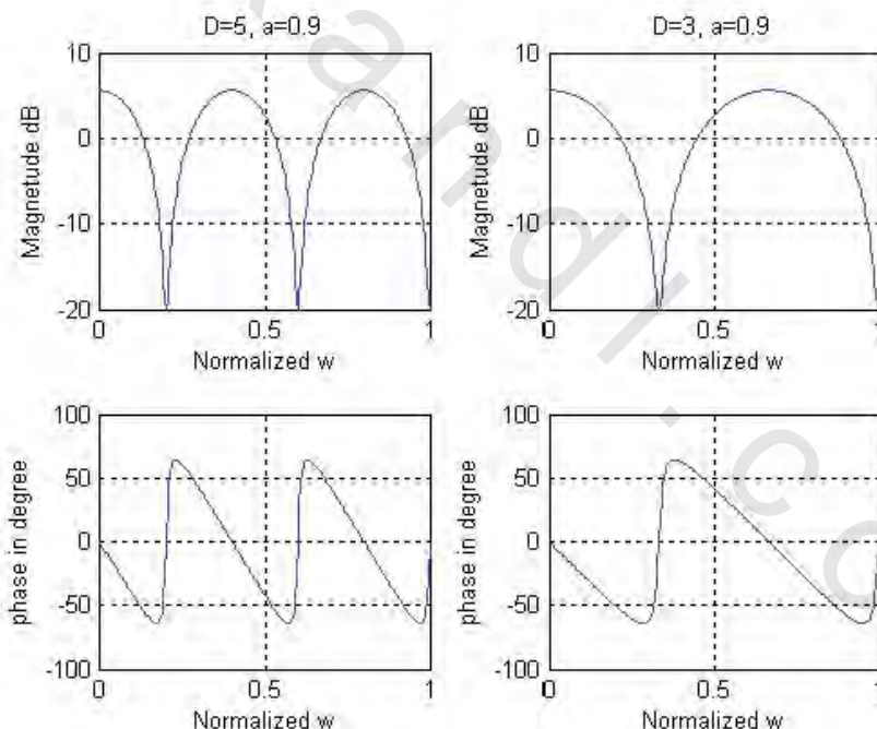
الشكل رقم (١٠، ١٠). الاستجابة الترددية لمروشح الصلدى الأحادي.
