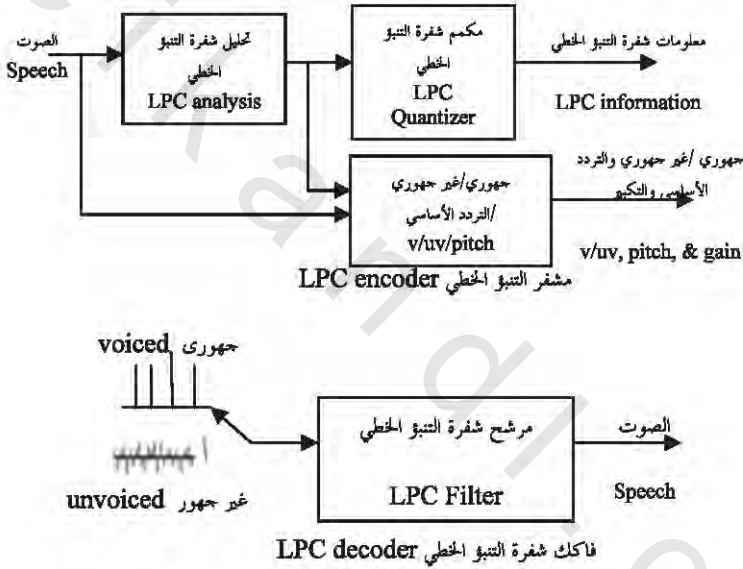
الشكل رقم (١٠.٥). تشفير الصوت وإعادة إنتاجه vocoder.
