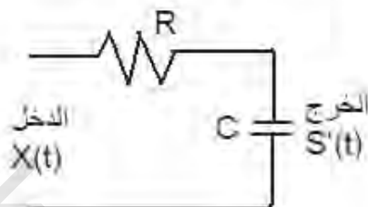
الشكل رقم (١.١). مرشح تناظري في أبسط صورة
