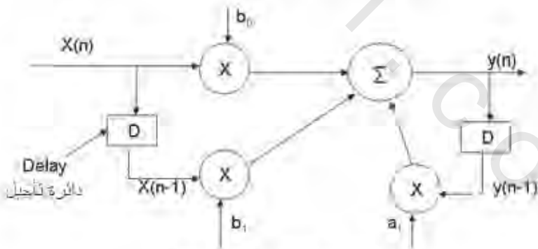
الشكل رقم (١.٣). بناء المرشح الرقمي .
