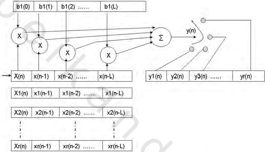
الشكل رقم (١.٦). ترشيح عدة إشارات بنفس المرشح.
