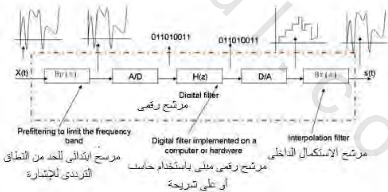
الشكل رقم (١.٢) رسم صندوق لنظام معالجة رقمي للإشارات.
