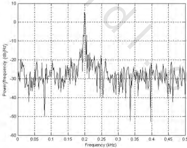
الشكل رقم (١.٩). النطاق الترددي من تحليل طيفي لموجة جيبية ترددها ٢٠٠ هرتز مضافاً إليها ضوضاء.
