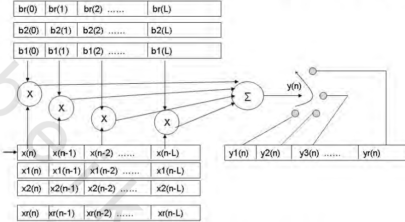
الشكل رقم (١.٧). عدة مرشحات لعدة إشارات.
