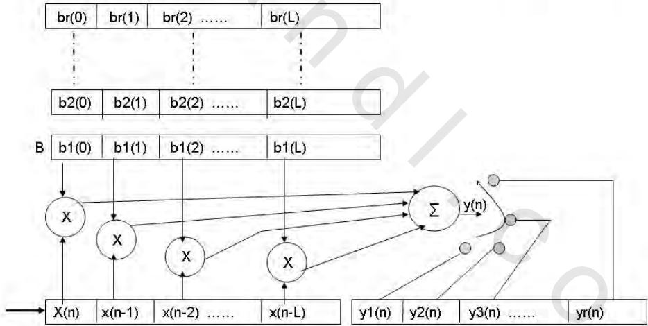
الشكل رقم (١,٥). عدة مرشحات لنفس الإشارة.
