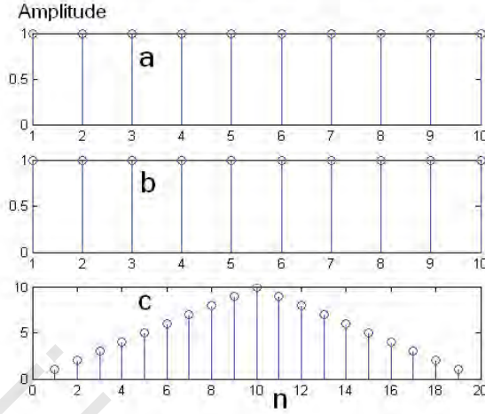
الشكل رقم (٣.٢٨). المجموع الالتفافي للتابعين.
