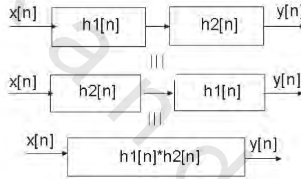
الشكل رقم (٣،٢٦). توصيل نظامين خطيين على التوالي.
