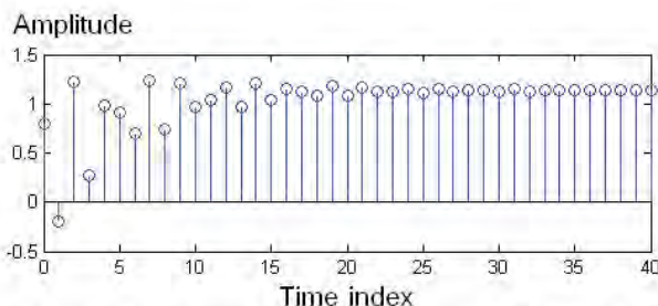
الشكل رقم (٣.٣٠). حساب استجابة الخطوة لنظام المعادلة رقم (٣.٤٤).
