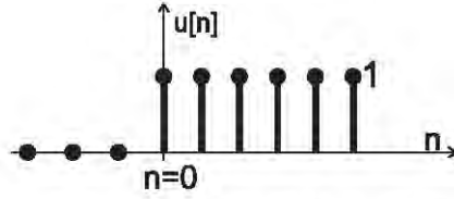
الشكل رقم (٣,٦). إشارة الدرجة الواحدة.
