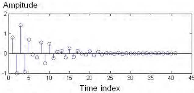
الشكل رقم (٣.٣١): حساب استجابة الصدمة باستخدام الدالة \text{impz} .
