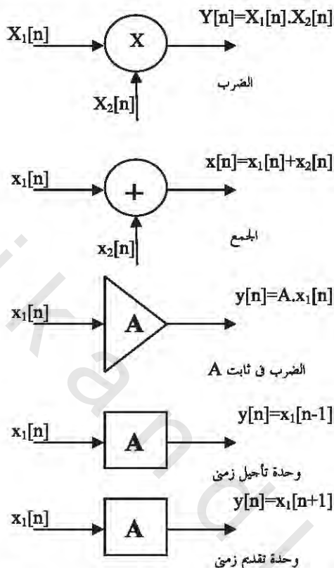
الشكل رقم (٣.١٤). العمليات الأساسية على المتتابعات.
