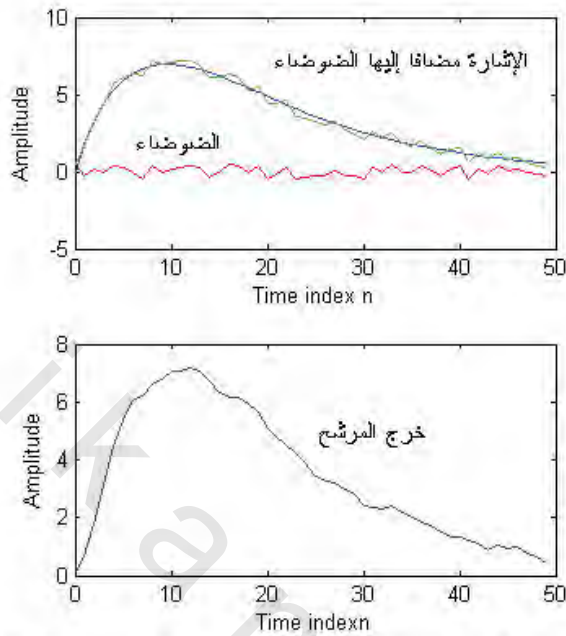
الشكل رقم (٣،١٨). مرشح نافذة المتوسط وتأثيره على الضوضاء، مثال رقم (٣،٤).
