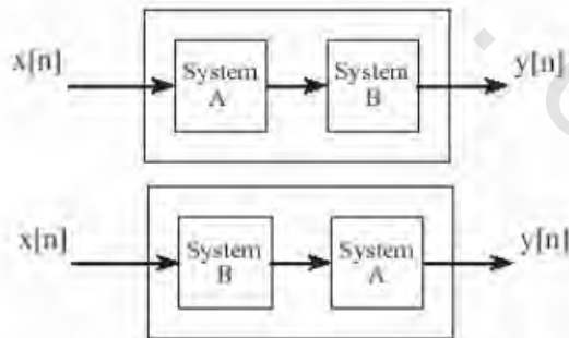
الشكل رقم (٣،١٩). خاصية المبادلية في الأنظمة الخطية.
