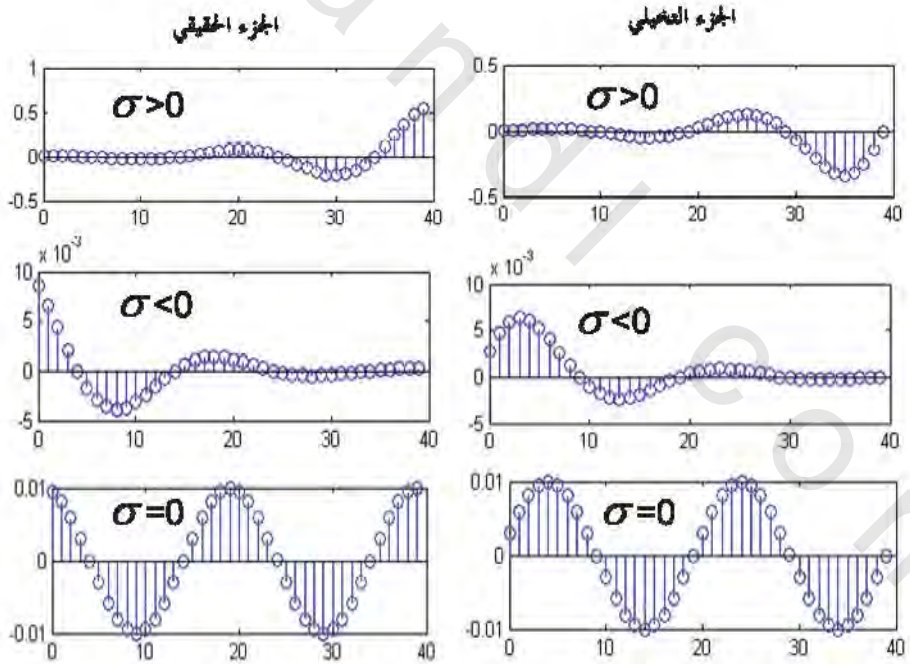
الشكل رقم (٣.٩). الجزء التخيلي والحقيقي عند قيم مختلفة للثابت \sigma في المعادلة رقم (٣.٨).
