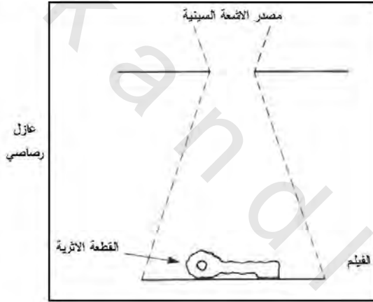
الشكل رقم (٤، ٣). نتاج ظلال التصوير بالأشعة.
