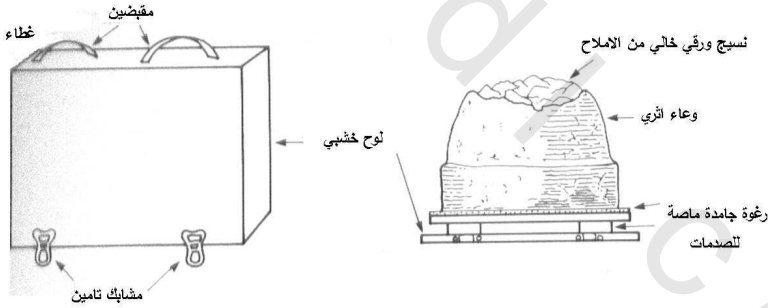
الشكل رقم (٣،٩). تغليف جرة من الفخار للتخزين والنقل.
