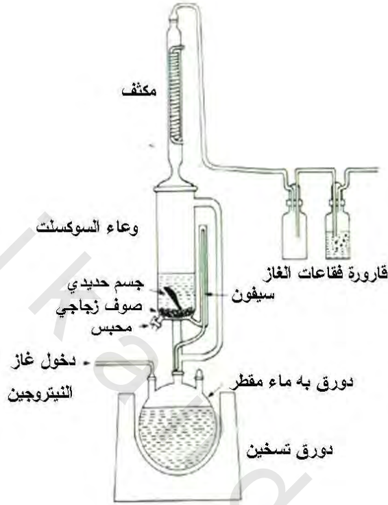
الشكل رقم (٣,١١). يستخدم مستخلص سوكسلت (Soxhlet) في جو خال من الأوكسجين. تزال الأملاح من مادة حديدية متأكلة تحت غاز النيتروجين (وفقاً لسكوت وسيلي: المرجع ٣٨، الفصل ٥).
