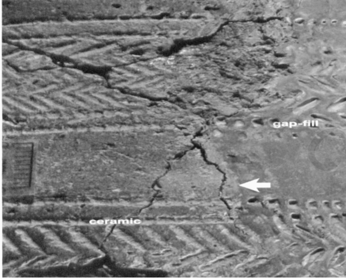
اللوحة (١٧، ٣). تشقق في سيراميك (منخفض الحرارة)، حدث بسبب انكماش مادة مائلة للنفجوات. يوضح السهم المكان الذي التصقت فيه تلك المادة بالإناء.
