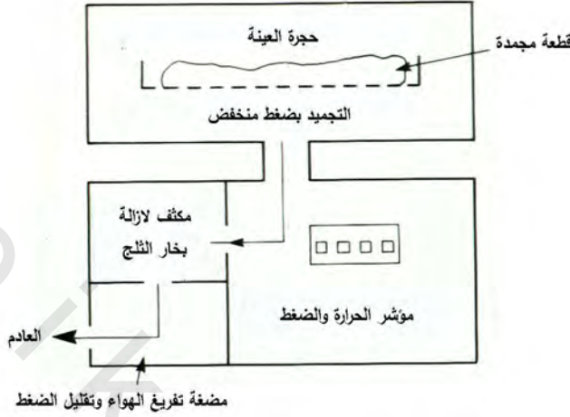
الشكل رقم (١٠، ٣). وظيفة المجفف - المبرد.
