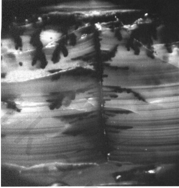
اللوحة (٤, ١١). صورة مجهرية فوتوغرافية لمقطع عرضي لقطعة من الزجاج النالف تبين طبقة القشرة المتعوية، من المحتمل أن تكون الريش المسوذة نتيجة لأكسدة الحديد والمانجنيز في الزجاج.
