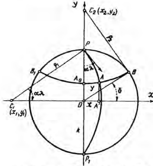
الشكل رقم (١٢٩). الشبكة في إسقاط لاغرانج.
