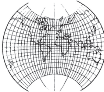
الشكل رقم (١٣٠). إسقاط (لاجرانج) لتمثيل منطقة العالم.
