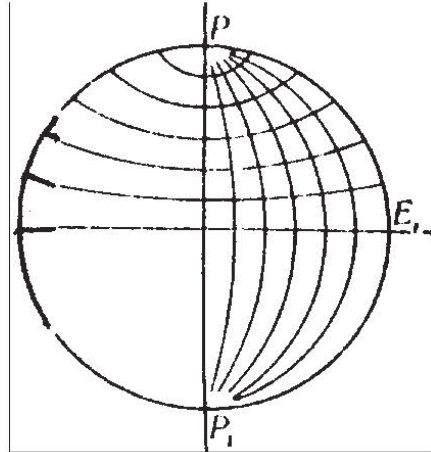
الشكل رقم (١٢٨). الشبكة في الإسقاط الكروي.
