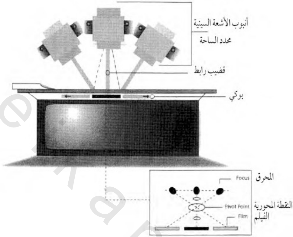
الشكل رقم (٤١). طاولة التصوير المقطعي.
