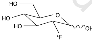
الشكل رقم (٢-٢). جزيئات مادة الفلوروديكسوجلوكون.
