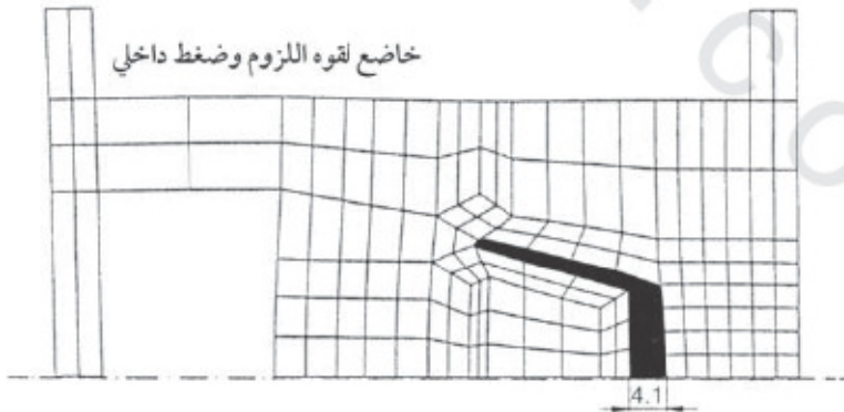
الشكل رقم (٨,٧). محاكاة خواص التشوه.
