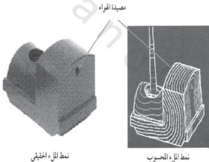
الشكل رقم (٨,٣). نمط التعبئة في لعبة القاطرة.
