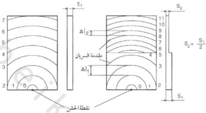
الشكل رقم (٨،٢). تأسيس أنماط التعبئة لقالبين بسيطين على هيئة صفائح.
