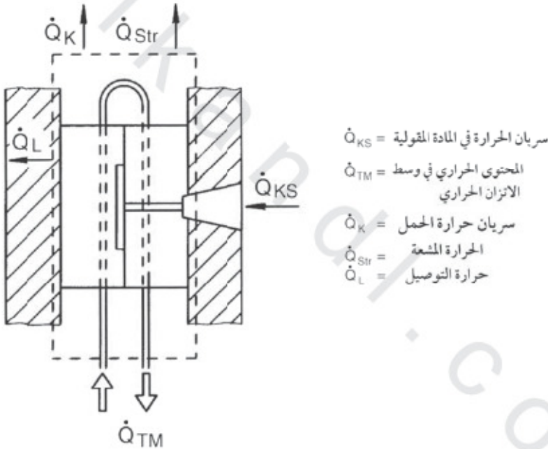
الشكل رقم (٨،٥). ميزان الحرارة لأداة القولية بالحقن.
