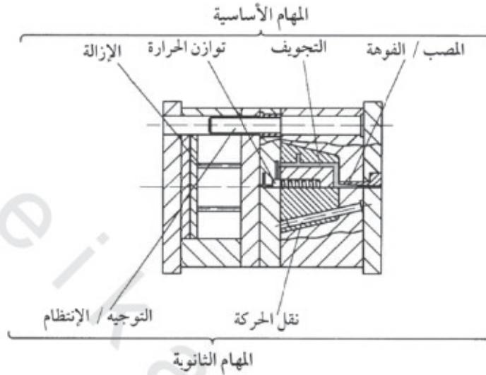
الشكل رقم (٨، ١). وظائف أداة القوالب بالحقن (قالب الانفصال).
