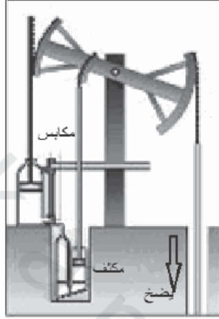
الشكل رقم (٥,٥). محرك واط.
