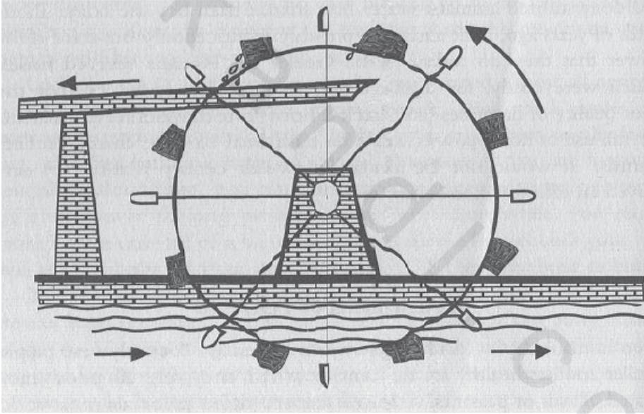
الشكل رقم (٥,١). الناعورة.
