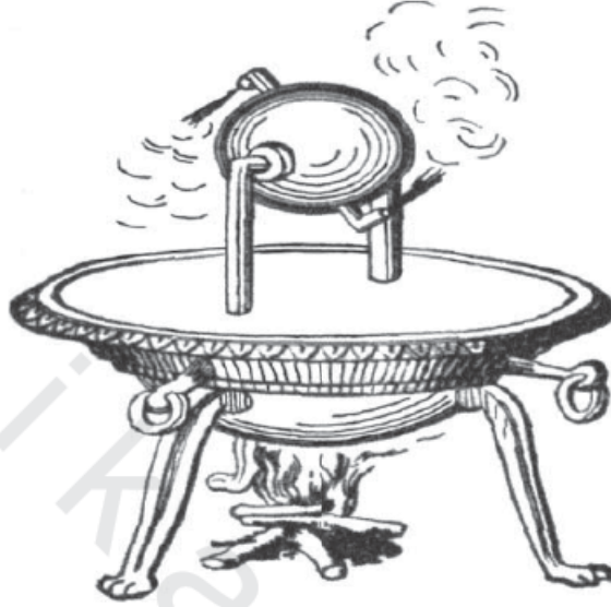
الشكل رقم (٥,٣). محرك هيرو.
