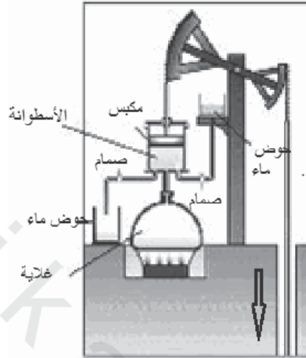
الشكل رقم (٤, ٥). محرك نيوكومين.
