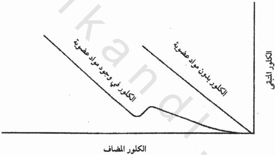
الشكل رقم (٦٧). منحني يوضح الطلب على الكلور، والكلور المتاح.
