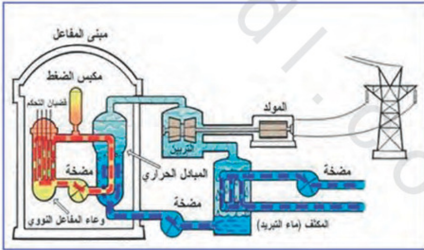
الشكل رقم (٢,٥). مفاعل الماء المضغوط (PWR) [٣٤].
