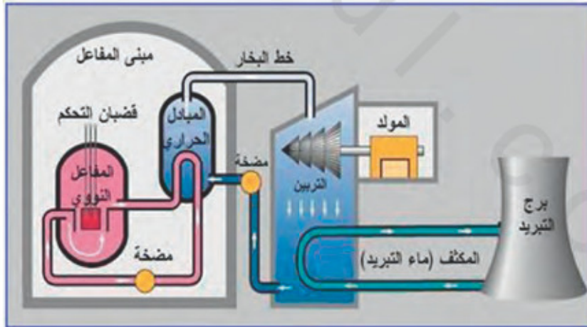
الشكل رقم (٢,١). نموذج محطة القدرة النووية.
