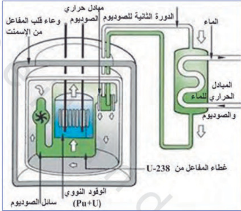
الشكل رقم (٢,٩). المفاعلات المولدة السريعة (FBR) [٣٧].
