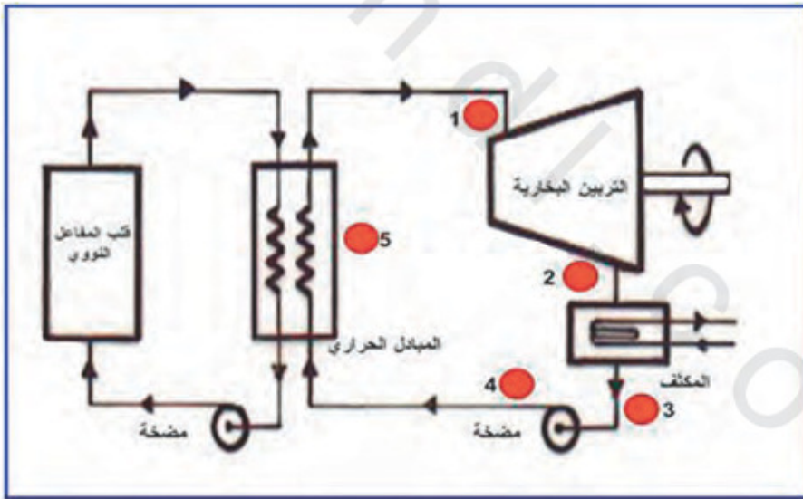
الشكل رقم (٢،٣). الخطوات الأساسية لتحويل الطاقة الحرارية إلى طاقة ميكانيكية في محطات القدرة النووية [٢].
