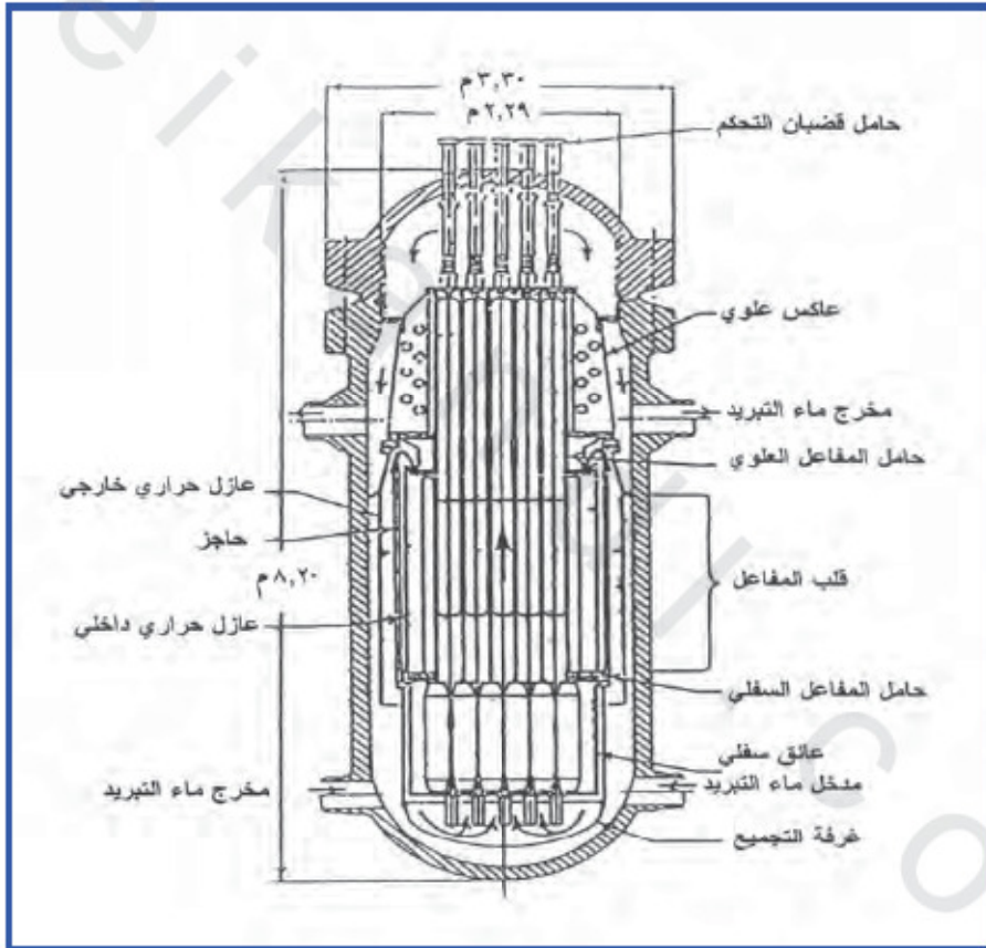
الشكل رقم (٢،٢). وعاء لمفاعل الماء المضغوط [٢].
