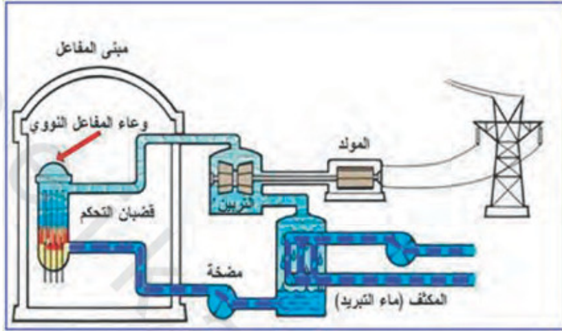
الشكل رقم (٢,٦). مفاعل الماء المغلي (BWR) [٣٤].
