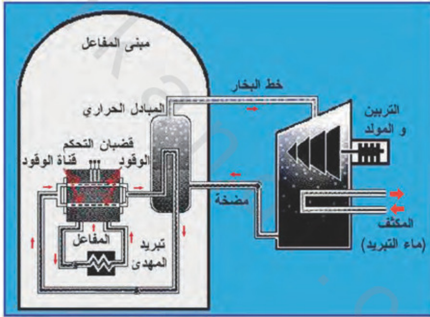
الشكل رقم (٢،٧). مفاعل الماء الثقيل المضغوط (PHWR) [٢٥].
