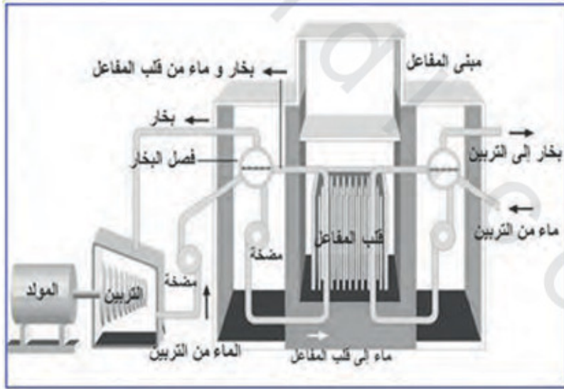
الشكل رقم (٢,٨). مفاعل الماء الخفيف والجرافيت (RBMK) [٢٩].
