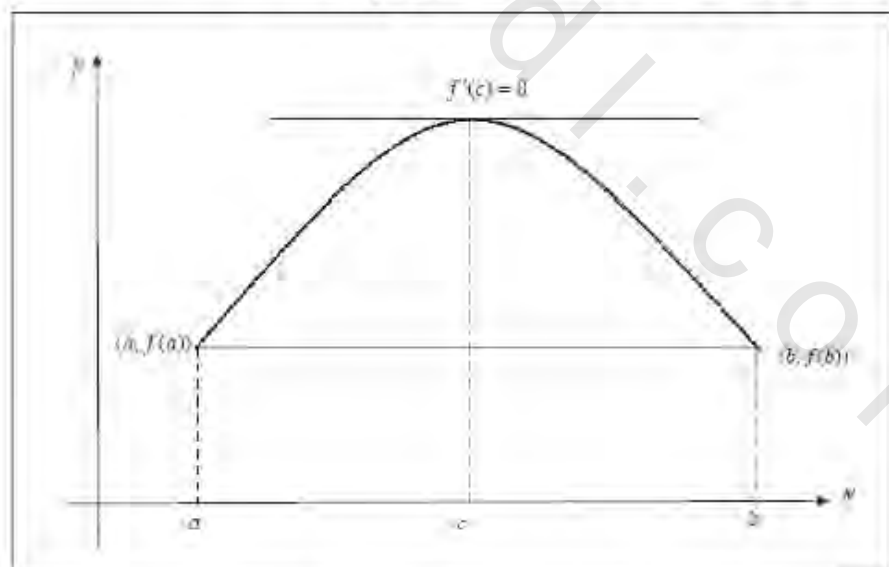
الشكل رقم (١،٢). شكل توضيحي لنظرية رول.
