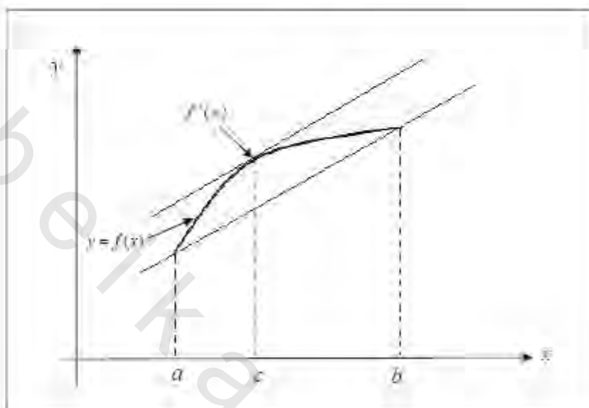
الشكل رقم (١,٣). شكل توضيحي للنظرية (١,٧).
