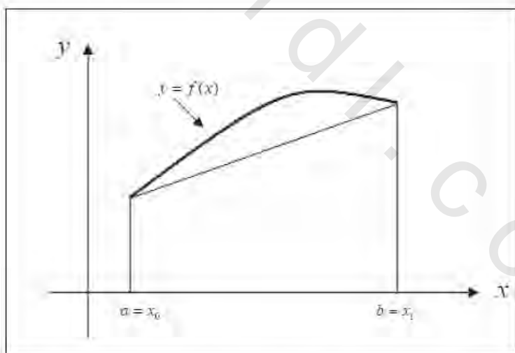
الشكل رقم (٥، ٢). صيغة شبه المنحرف عندما f(x) \geq 0 .
