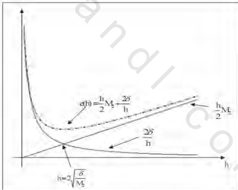
الشكل رقم (٥، ١). نمو الخطأ على طرفي القيمة المثلى لـ h .
