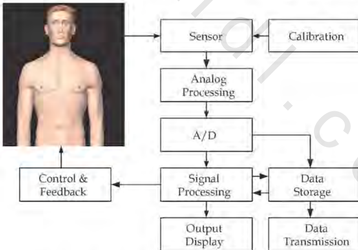
الشكل رقم (٢.٩). الأنظمة الأساسية للتجهيزات باستخدام الحساسات لقياس إشارة مع إمكانيات اقتباس البيانات وتخزينها وعرضها، بالإضافة إلى التحكم والتغذية العكسية.
