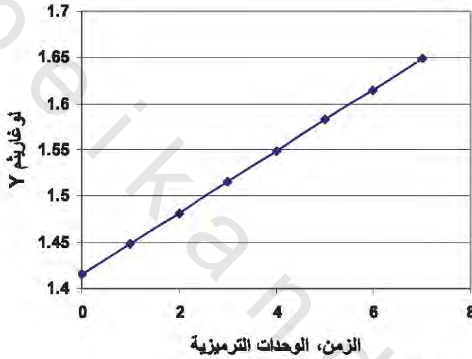
الشكل رقم (١١.٥). تمثيل الخط للاتجاه غير الخطي.
