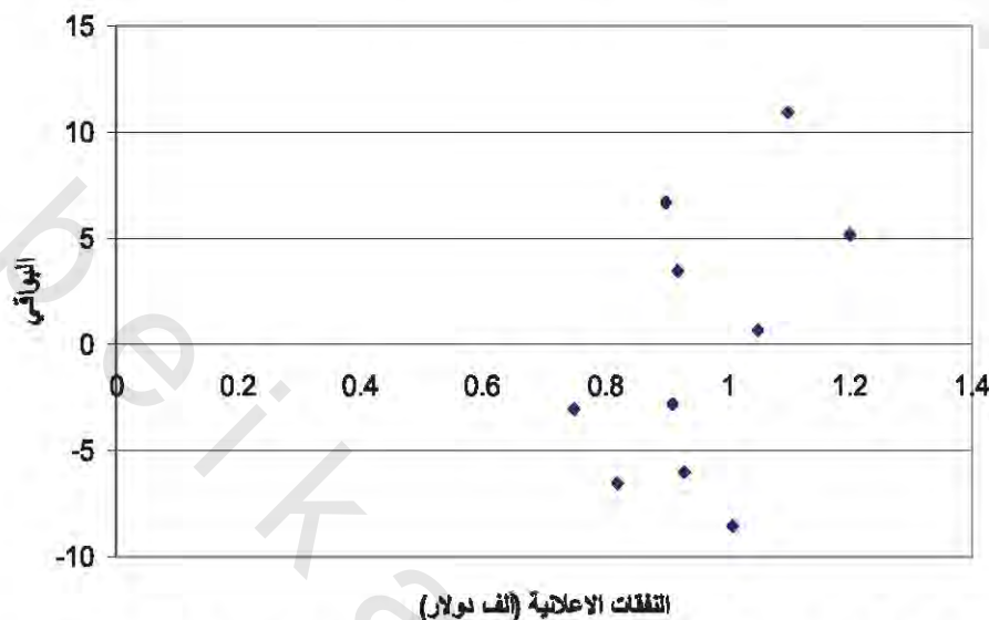
الشكل رقم (١١.٣). شكل الانتشار للبواقى من نموذج الانحدار للتفقات الاعلانية والمبيعات الشهرية.
