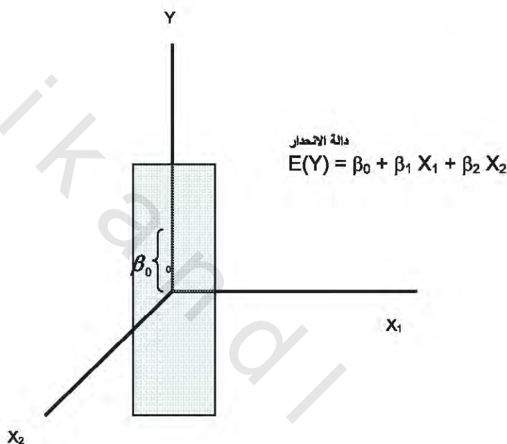
الشكل رقم (١١.٤). مسطح دالة الانحدار في حالة متغيرين مستقلين.
