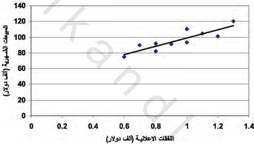
الشكل رقم (١١.٢). تقدير خط الانحدار لبيانات الإعلان والمبيعات للمحل الزراعي.
