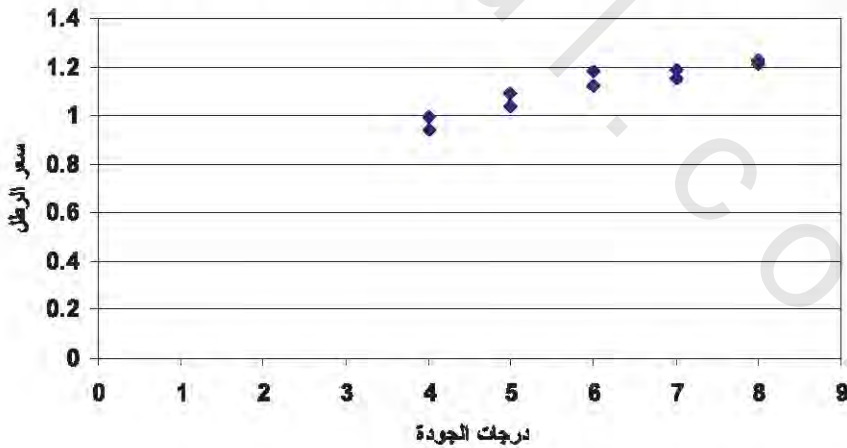
الشكل رقم (١١.١). شكل الانتشار لبيانات شرائح ثور لانيوس.
