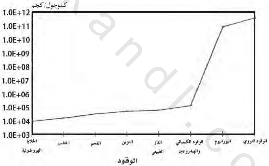
الشكل رقم (١,٥). التسلسل التاريخي لاستغلال الطاقة كدالة في الطاقة النوعية.
