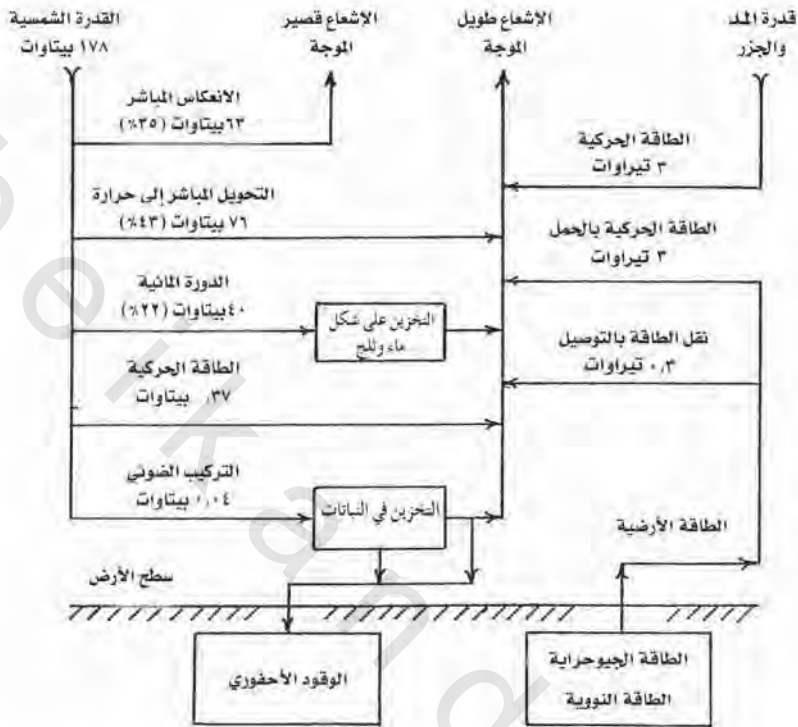
الشكل رقم (٢,١). رسم تخطيطي لتدفق الطاقة على الأرض.
