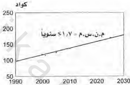
الشكل رقم (٤، ٣). استهلاك الطاقة التاريخي والمقدر في الولايات المتحدة منذ ١٩٩٠ - ٢٠٢٥م [3].
