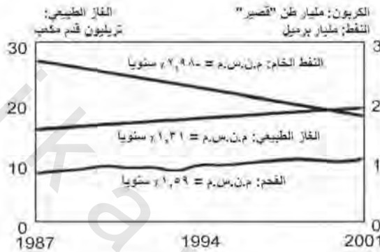
الشكل رقم (٣,٣). إنتاج الوقود الأحفوري في الولايات المتحدة منذ ١٩٨٧ - ٢٠٠١ م [3].
