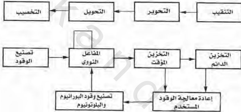
الشكل رقم (٦,٧). دورة وقود اليورانيوم لمفاعلات الماء الخفيف النووية.
