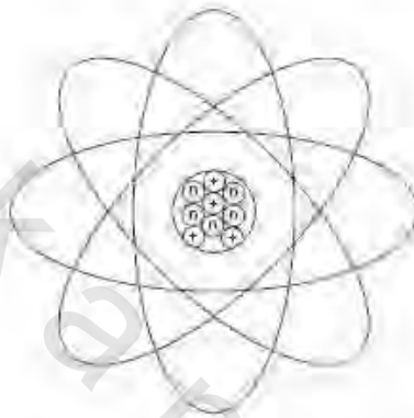
الشكل رقم (٦، ١). نموذج هندسي لنواة الذرة مع الإلكترونات المحيطة بها.
