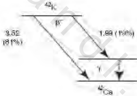
الشكل رقم (٦، ٤). طريقة التحلل للنظير المشع البوتاسيوم-٤٢ ( ^{42}\text{K} ).
