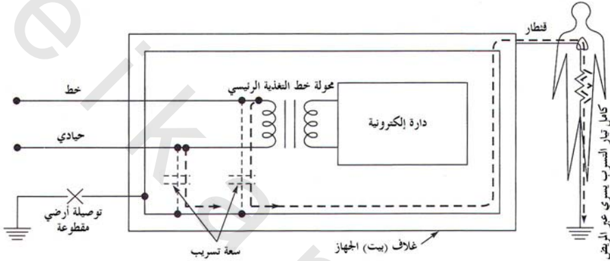
الشكل رقم (١٨,٨). مسار تيار التسريب حالة عدم استمرارية الأرضي (معد ر ه وافقة شركة Hewlett Packard).
