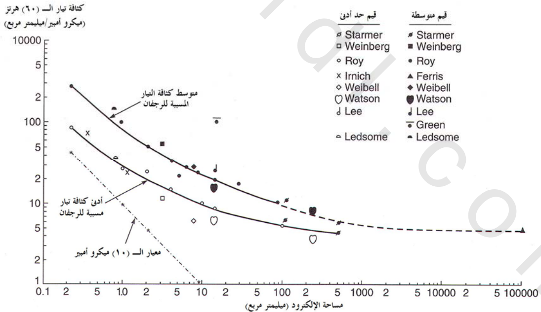
الشكل رقم (١٨،٤). العلاقة بين كثافات التيار المسببة للرجفان كتابع مساحة الإلكترود (حسب Roy (1980)، معاد إنتاجه وألفه Med. & Biol. Eng. & Comput.).
