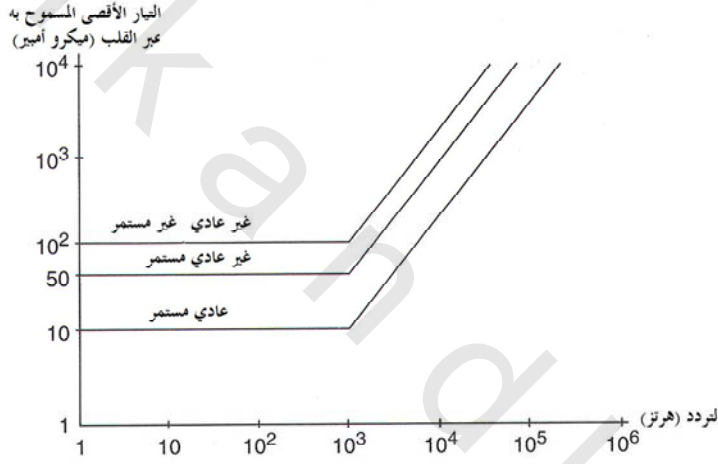
الشكل رقم (١٨,٢). تيار التسرب الأقصى المسموح به عبر القلب كتابع للتردد ( وافقه Philips Medical Systems ).
