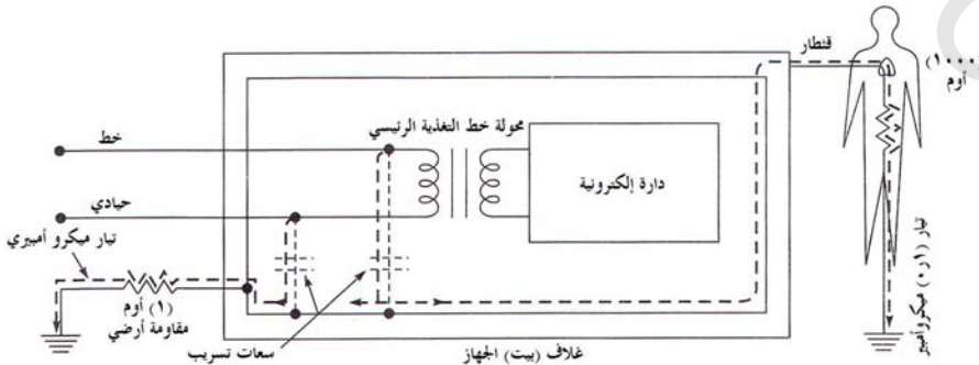
الشكل رقم (١٨,٧). مسار تيار التسريب حالة عادية x أن سلك التأريض سليم (معد ر ه وافقة شركة Hewlett Packard).
