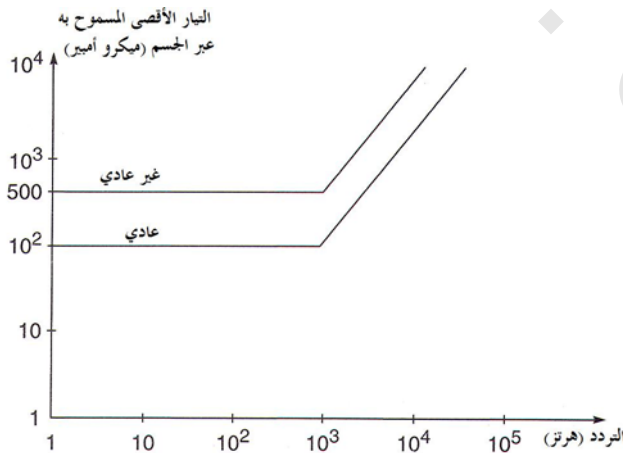
الشكل رقم (١٨، ١). تيارات التسرب القصوى المسموح بها | اسم كيناي للتردد (وافقه Philips Medical Systems).
