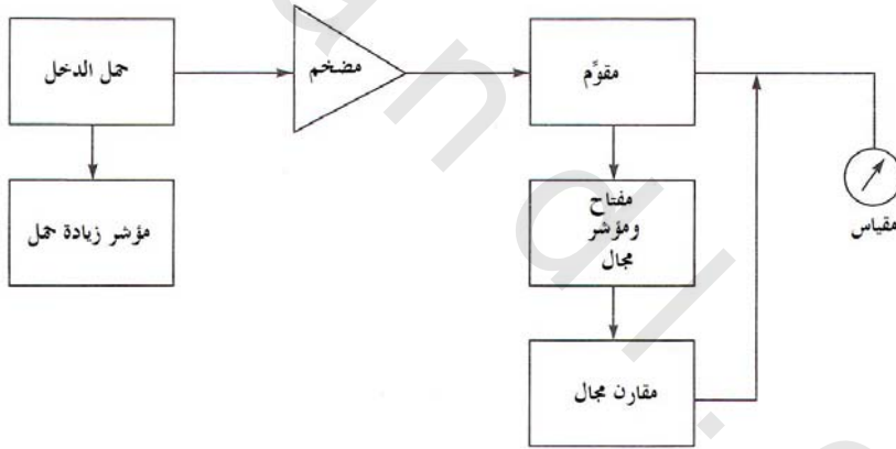
الشكل رقم (١٨,٩). رسم مخطط قياس تيار التسريب.
