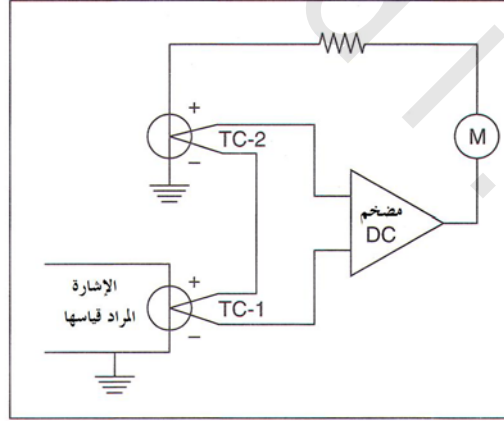
الشكل رقم (٢٧، ١١). مبدأ عمل جهاز لبل الإنفاذ ا راري.
