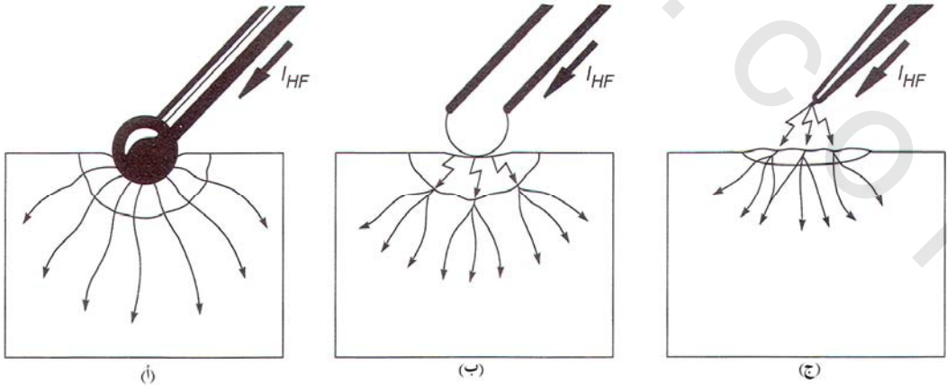
الشكل رقم (٢٧, ٧). (أ) طري. (ب) قسري. (ج) بالتبريق.
