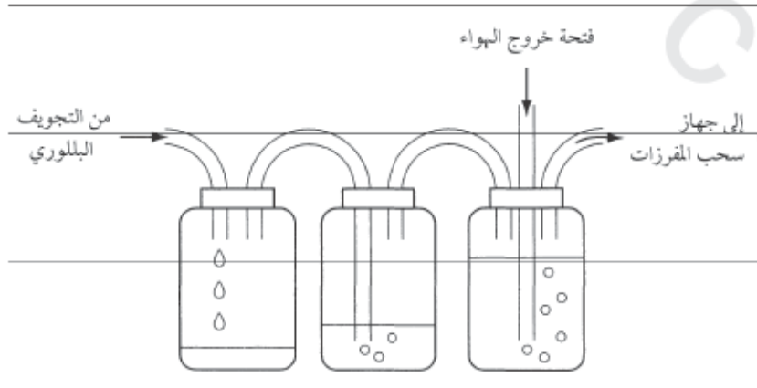
الشكل رقم (١). جهاز تصريف السوائل ثلاثي الحجرات.
