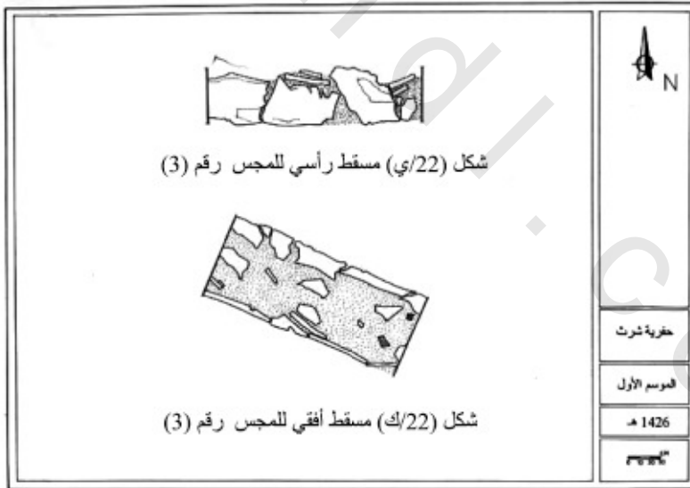
الشكل رقم ( ٢٢ ي، ك). المذيل الحجري رقم (٢) مسقط رأسي ومسقط أفقي للمجس رقم (٣). المصدر : من عمل الباحثين.
