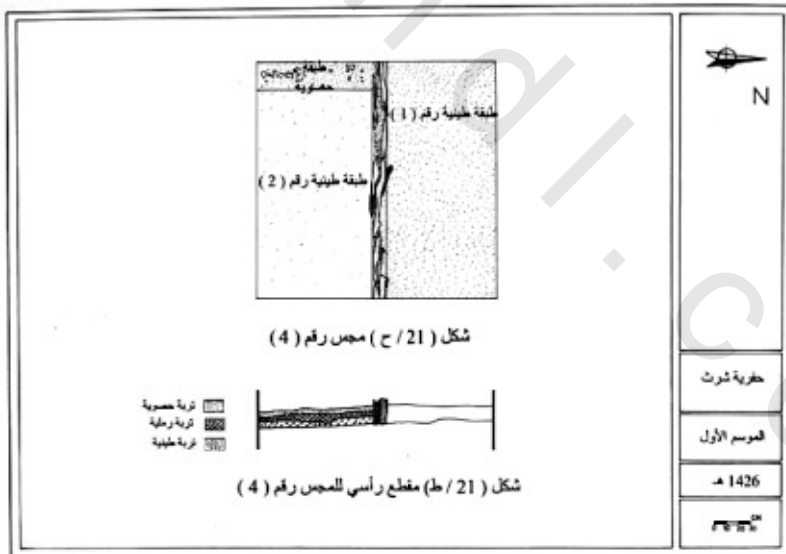
الشكل رقم ( ٢١ ح ، ط ) . المذيل الحجري رقم ( ١ ) : مجس ( ٤ ) مقطع رأسي للمجس رقم ( ٤ ) .
