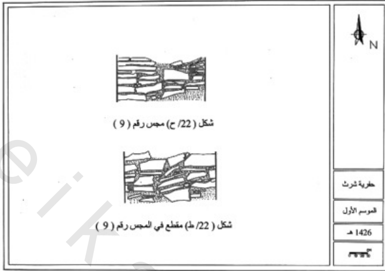
الشكل رقم ( ٢٢ ح، ط). المذيل الحجري رقم (٢) مجس رقم (٩). المصدر : من عمل الباحثين.
