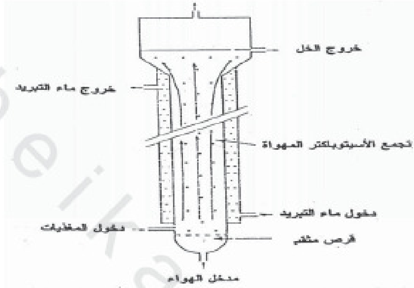
الشكل رقم (١١,٦). أحد أجهزة طريقة الغمر لتصنيع الخل (من نوع البرج).
