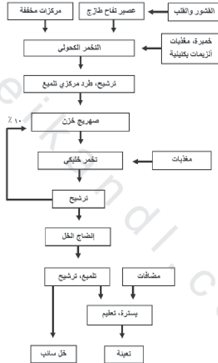
الشكل رقم (١١،٤). خطوات تصنيع خل التفاح.
