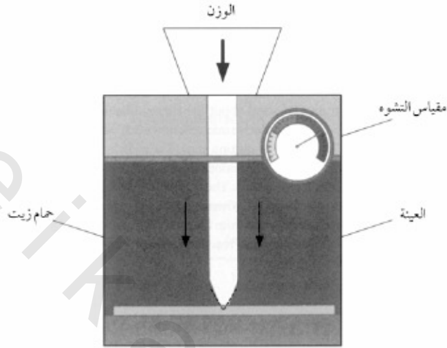
الشكل رقم (٤,٢). اختبار درجة حرارة ليونة فايكات.
