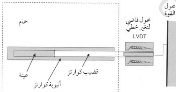
الشكل رقم (٤,٥). جهاز التمدد الخطي.
