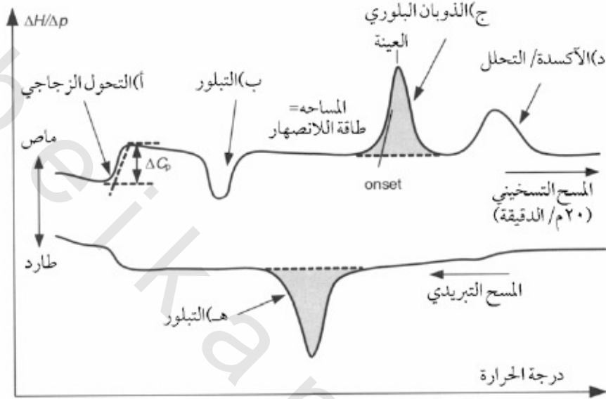
الشكل رقم (٤، ٤). رسم تمثيلي للتحويل الطارد والماص للحرارة من اختبار المسح التفاضلي المسعري.
