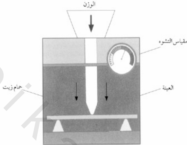
الشكل رقم (٤,١). اختبار حرارة التشكل.
