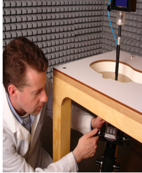
شكل (5 - 7) قياس معدل الامتصاص النوعي SAR عمليا
