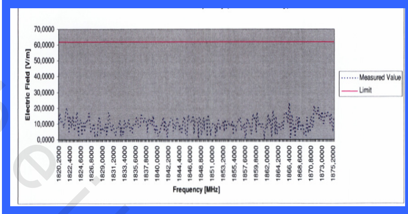
شكل ( 5 - 4 ) شدة المجال الكهربائي كدالة للتردد ( GSM 1800 )
