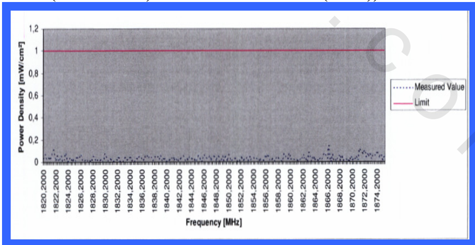
شكل ( 5 - 5 ) كثافة القدرة كدالة للتردد ( GSM 1800 )
