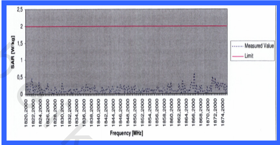
شكل ( 5 - 6 ) SAR كدالة للتردد ( GSM 1800 )
