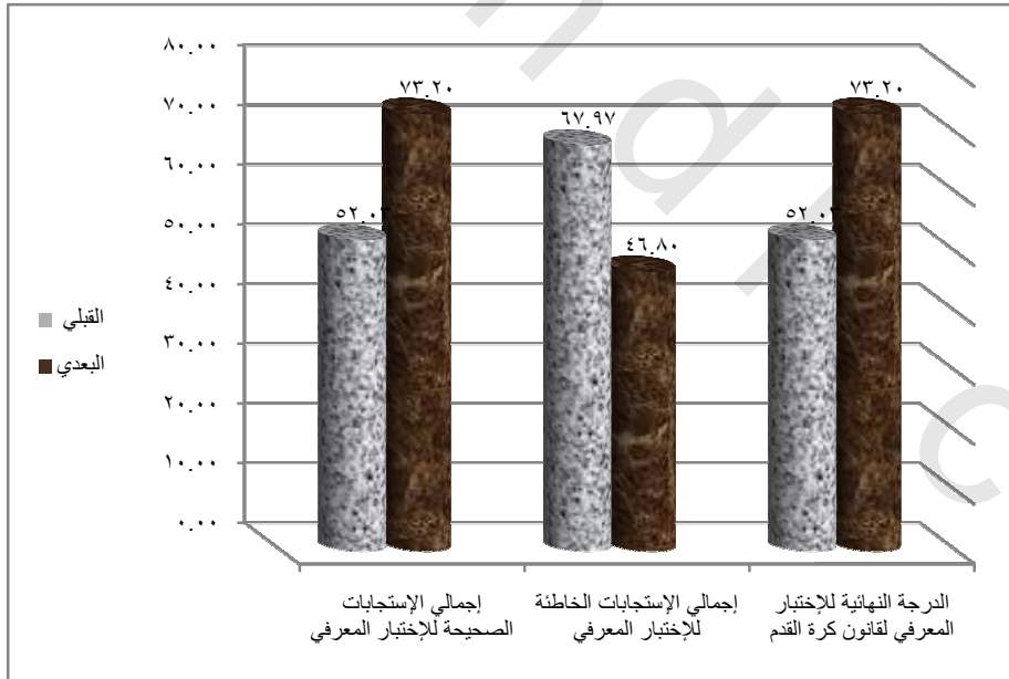
الشكل البياني (٦) يوضح الفرق بين القياسيين القبلي والبعدي في الإختبار المعرفي لقانون كرة القدم للمجموعة الضابطة
