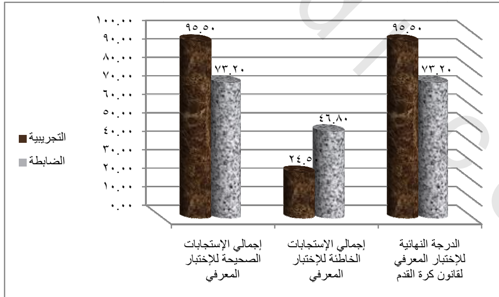
الشكل البياني (٧) يوضح الفرق بين القياسات البعدية في الاختبار المعرفي لقانون كرة القدم للمجموعتين التجريبية والضابطة
