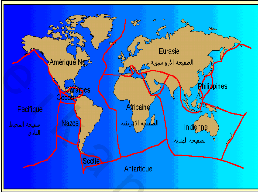
شكل ( ) الصفائح الصخرية في العالم .
