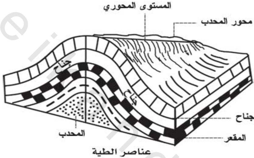
شكل ( ) يوضح مراحل تكوين الطية .
