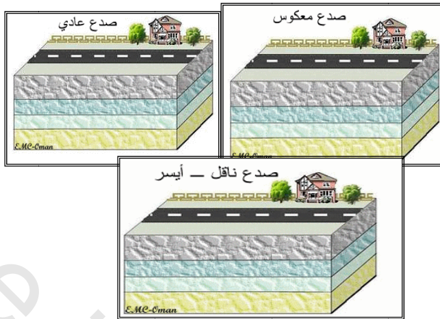
شكل ( ) يوضح مراحل تكوين الصدوع .
