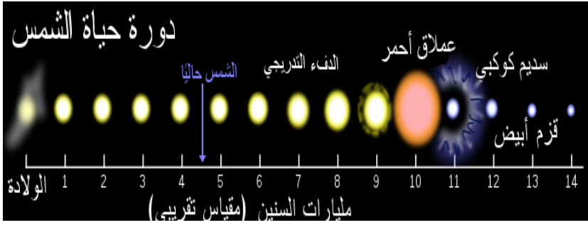
شكل ( ) يظهر دورة حياة الشمس .
