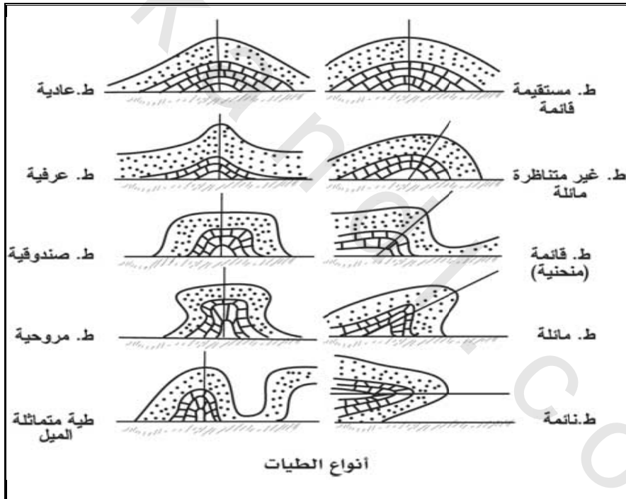
شكل ( ) يوضح أنواع الطيات .
