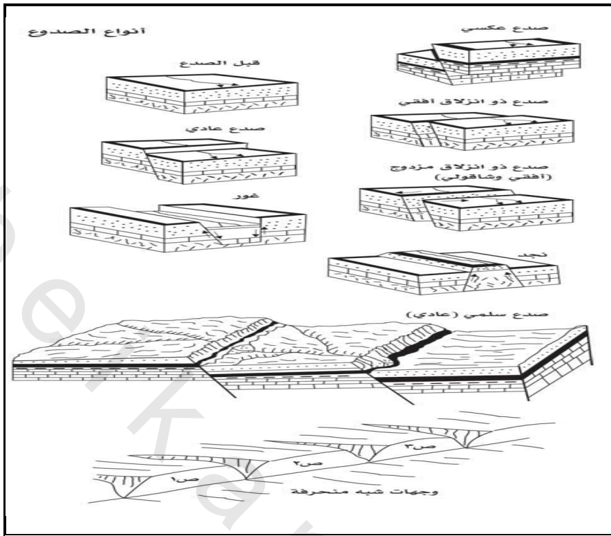
• شكل ( ) يوضح أنواع الصدوع .
