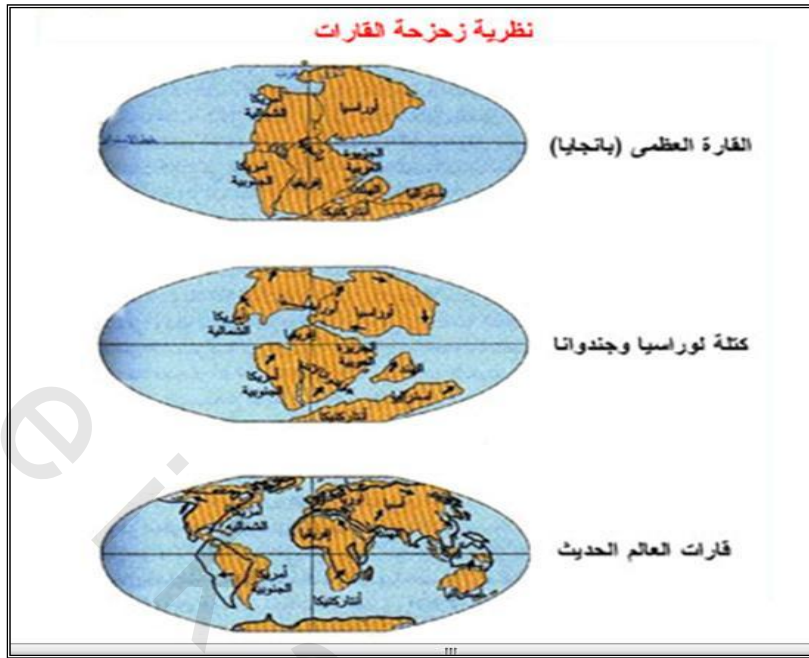
شكل ( ) نظرية زحزة القارات .
