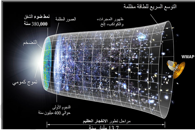
شكل ( ) يظهر مراحل تطور الانفجار العظيم .
