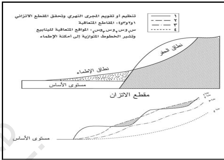
شكل ( ) يوضح نطاق الحفر والإطماء ومستوى الأساس .
