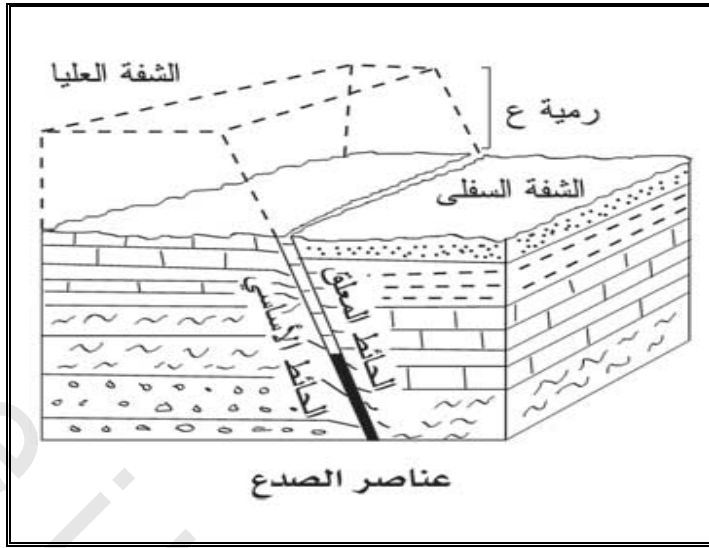
شكل ( ) يوضح عناصر الصدوع .
