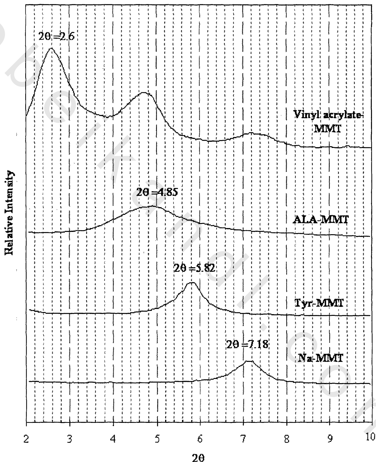
Figure 25: The X-ray diffraction patterns of Tyr-MMT ( I_0 ), ALA-MMT ( I_0 ), vinyl acrylate-MMT ( I_0 ) and Na-MMT
