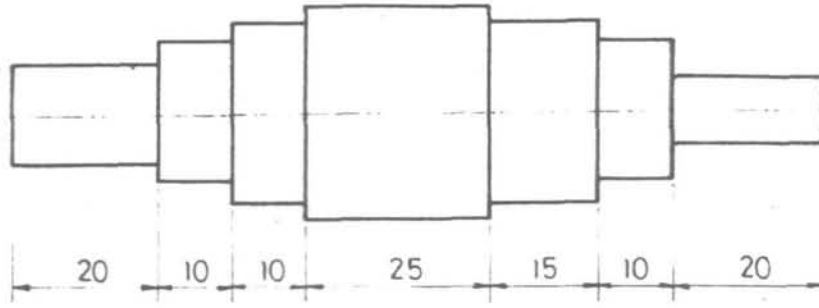
شكل « ٩ - ٨ » وضع الأبعاد بالطريقة التتابعية
