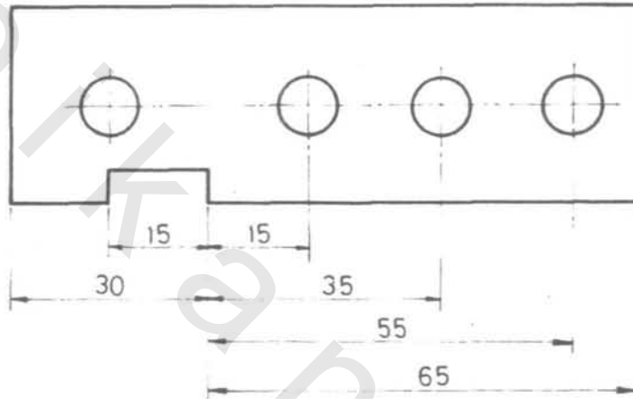
شكل « ٩ - ٩ » وضع أبعاد مقاسة من مرجع مشترك
