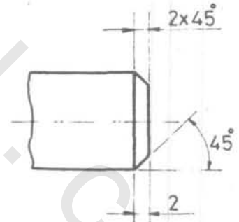
شكل « ٩ - ١٠ » أبعاد الشطفت
