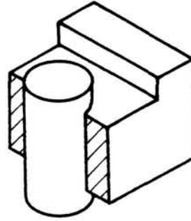
شكل « ٩-٨ » عدم تهشير مقاطع الأعمدة والبؤز
