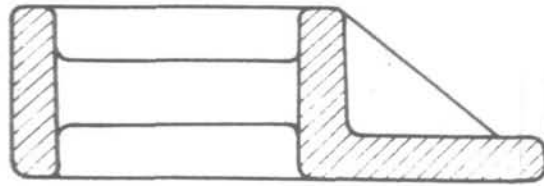
شكل « ٧-٨ » عدم تهشير أعصاب التقوية
