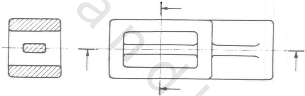
شكل « ٧-٨ » عدم تهشير أعصاب التقوية
