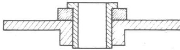
شكل « ٦-٨ » تهشير الأجزاء المتلاصقة
